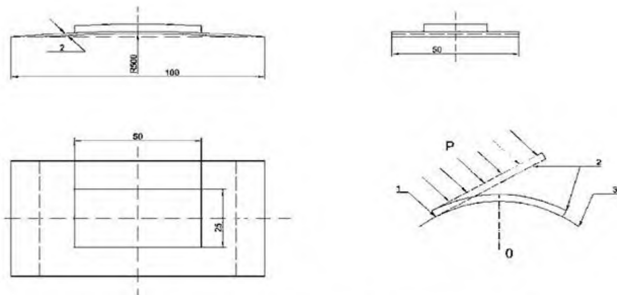
1 – отметка на шаблоне; 2 – образец-плитка; 3 – металлический шаблон
