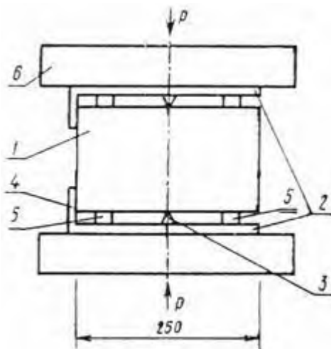
1 - образец; 2 - основание; 3 - металлический нож; 4 - упор; 5 - резиновые прокладки; 6 - плита пресса
