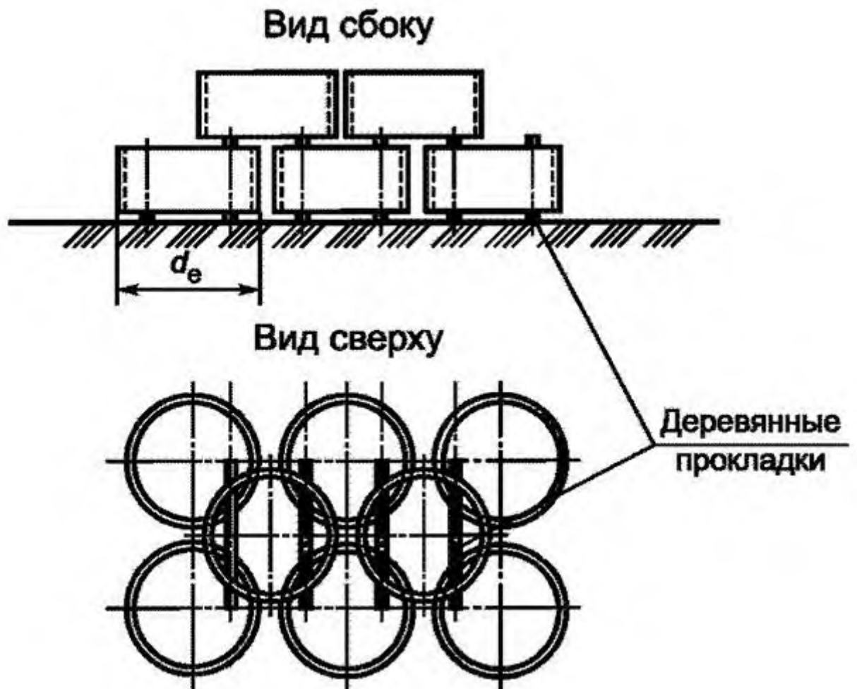
Рисунок 1 - Складирование стеновых колец колодцев
