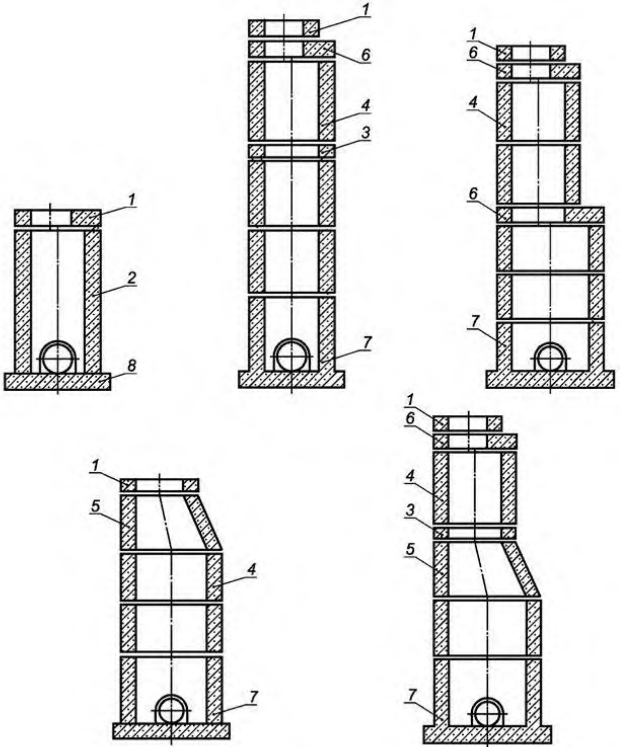
1 — плита перекрытия (дорожная); 2 — рабочая камера; 3 — опорное кольцо; 4 — стеновое цилиндрическое кольцо; 5 — стеновое коническое кольцо; 6 — опорная плита; 7 — стеновое кольцо с дном; 8 — плита дна
