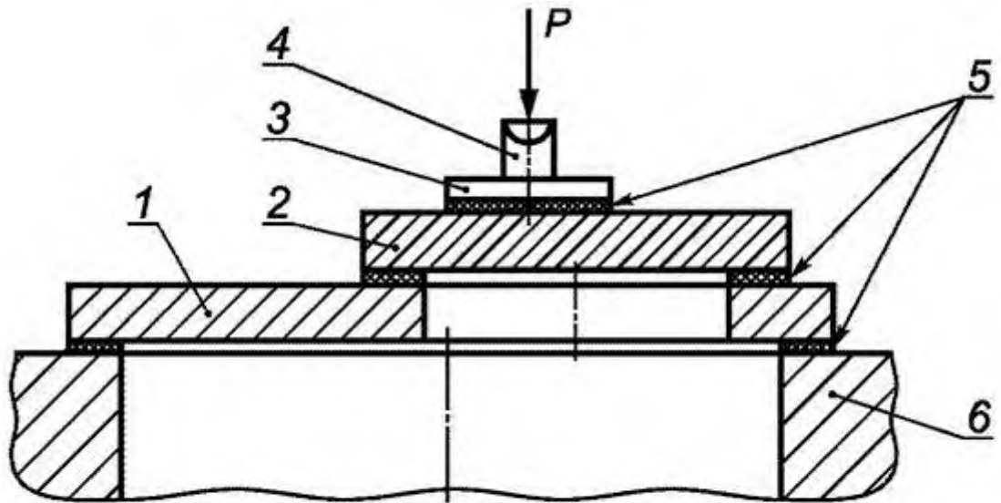
1— плита перекрытия; 2 — стальная плита; 3 — нагрузочная плита 300×300 мм; 4 — шаровая опора; 5 — резиновые прокладки; 6 — стеновое кольцо
