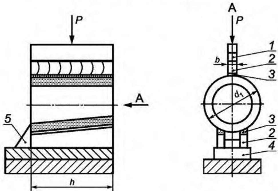
а) Цилиндрические стеновые кольца
