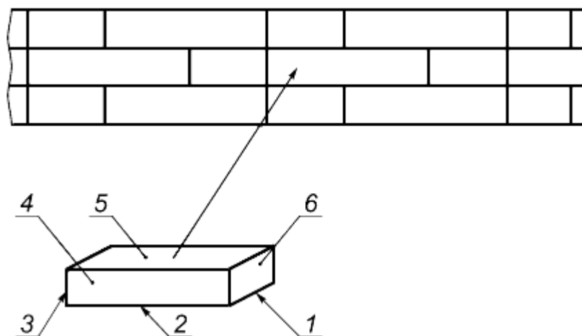
Рисунок 1 - Фрагмент кладки
