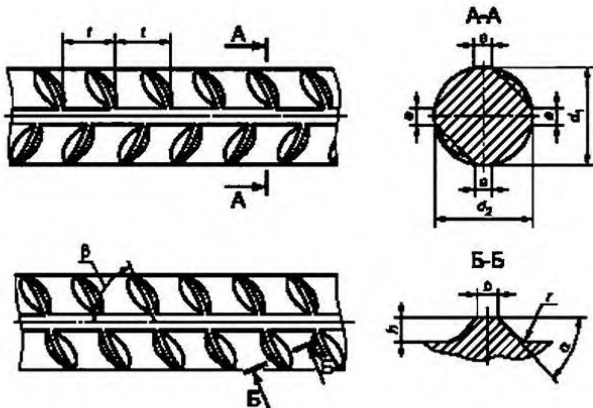
Рисунок 4 - Конфигурация и параметры периодического профиля по форме 4φ
