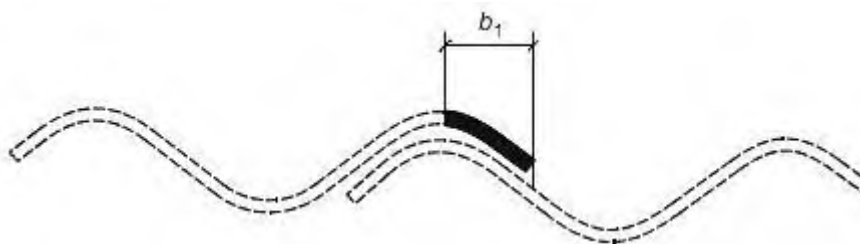
Рисунок 2 - Перекрывающаяся кромка листа
