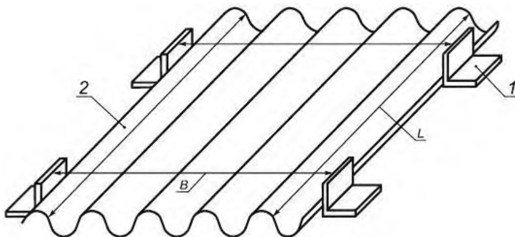
Рисунок 11 - Схема измерения размеров листов
