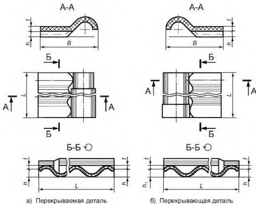
Рисунок 6 - Коньковые детали
