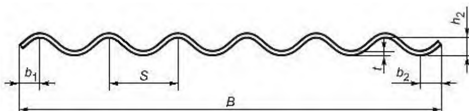
Рисунок 5 - Профиль листа 51/177 с асимметричными кромками
