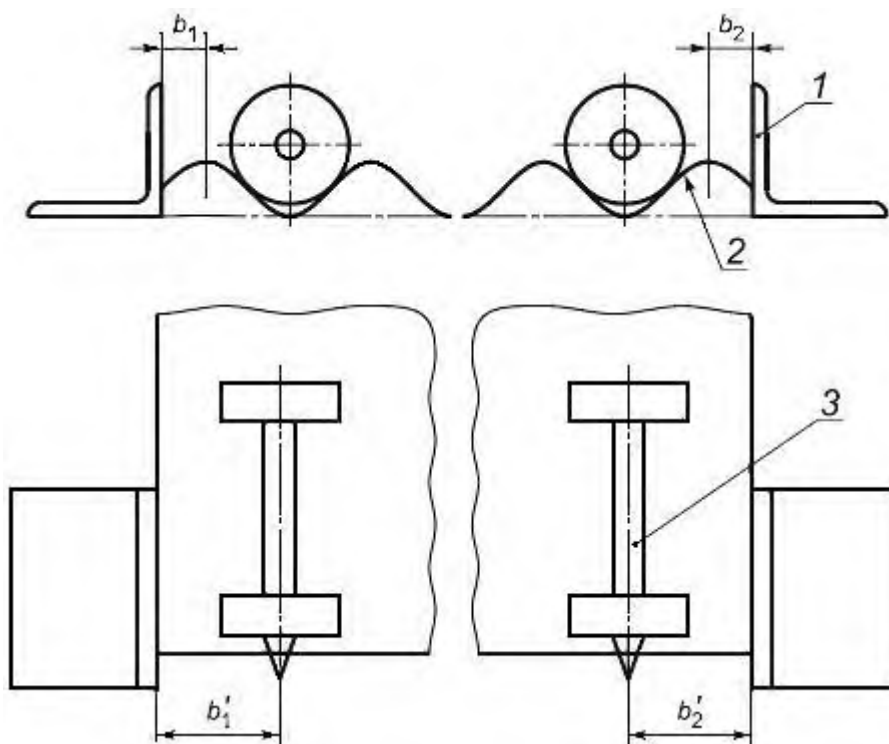
Рисунок 17 - Схема измерения ширины перекрывающей (перекрываемой) кромки
