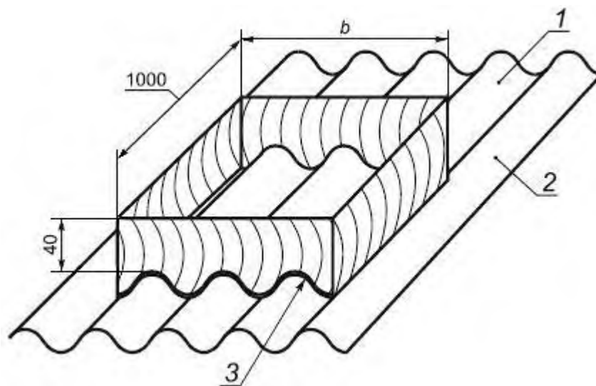
Рисунок 23 - Рама для определения водонепроницаемости
