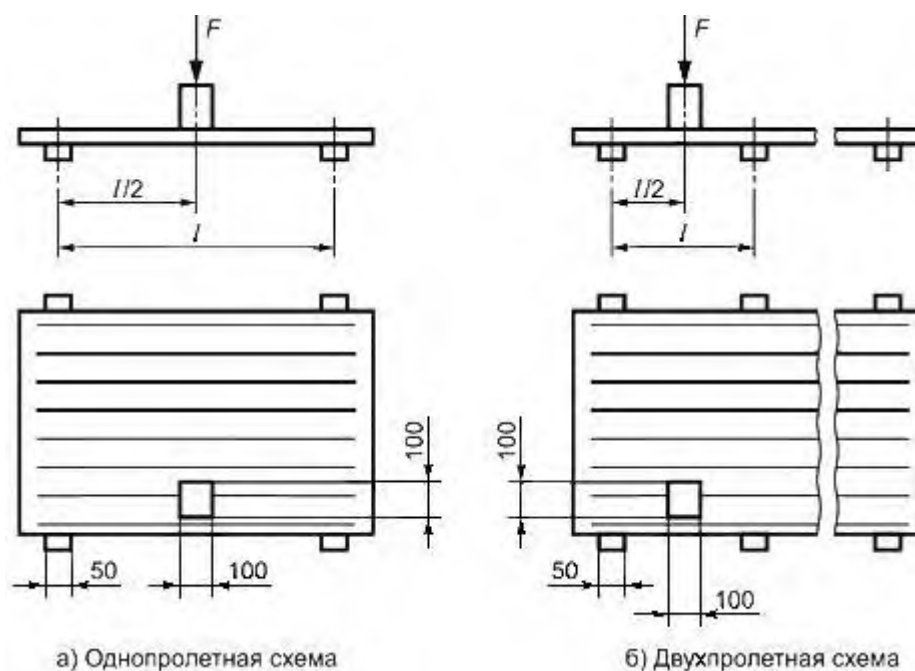
Рисунок 22 - Схемы испытания целых листов сосредоточенной штамповой нагрузкой
