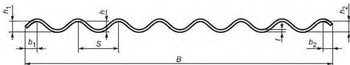
Рисунок 4 - Профиль листа 40/150 с симметричными кромками
