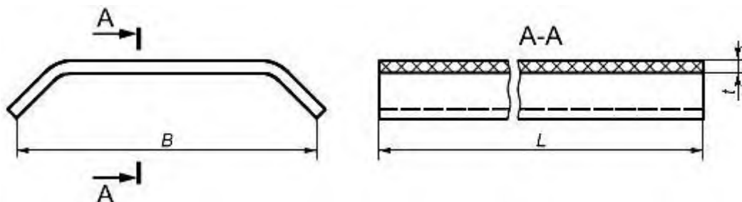
Рисунок 10 - Лотковая деталь
