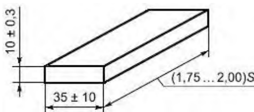
Рисунок 13 - Металлическая накладка для измерения высоты волны
