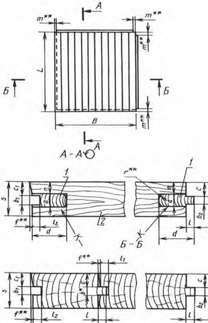
1 - шпонка; 2 - рейка Черт. 1
