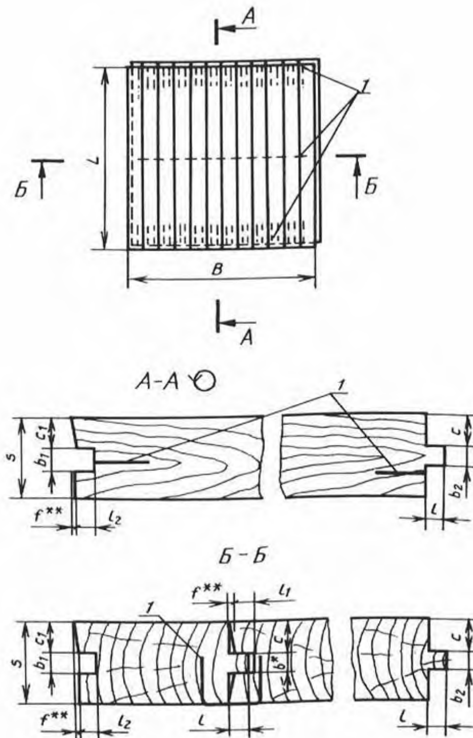
1 -скобы Черт. 2
