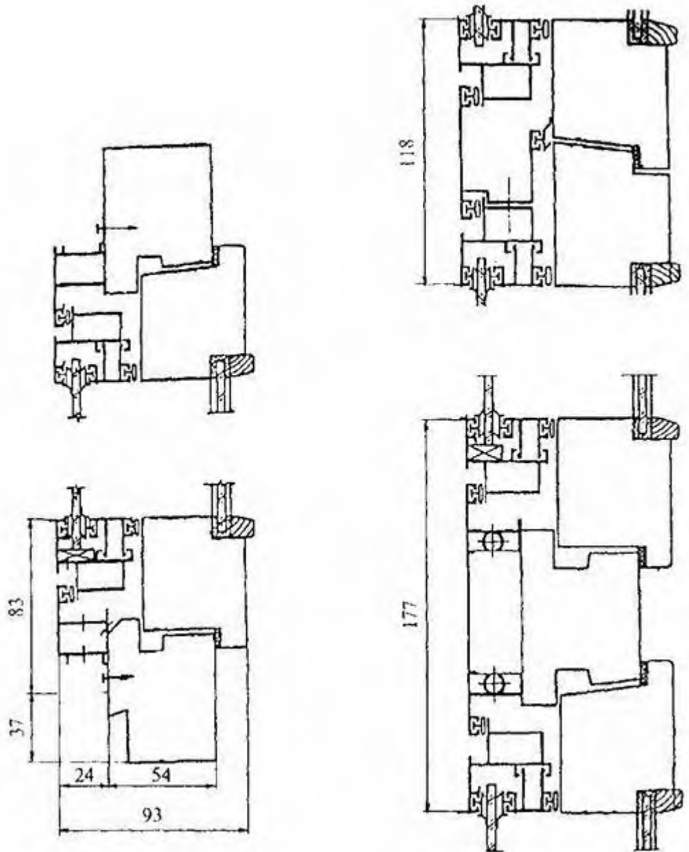
Рисунок 8 - Примеры конструктивных решений оконных блоков спаренной конструкции с алюминиевыми наружной створкой и коробкой и деревянными внутренними створкой и коробкой
