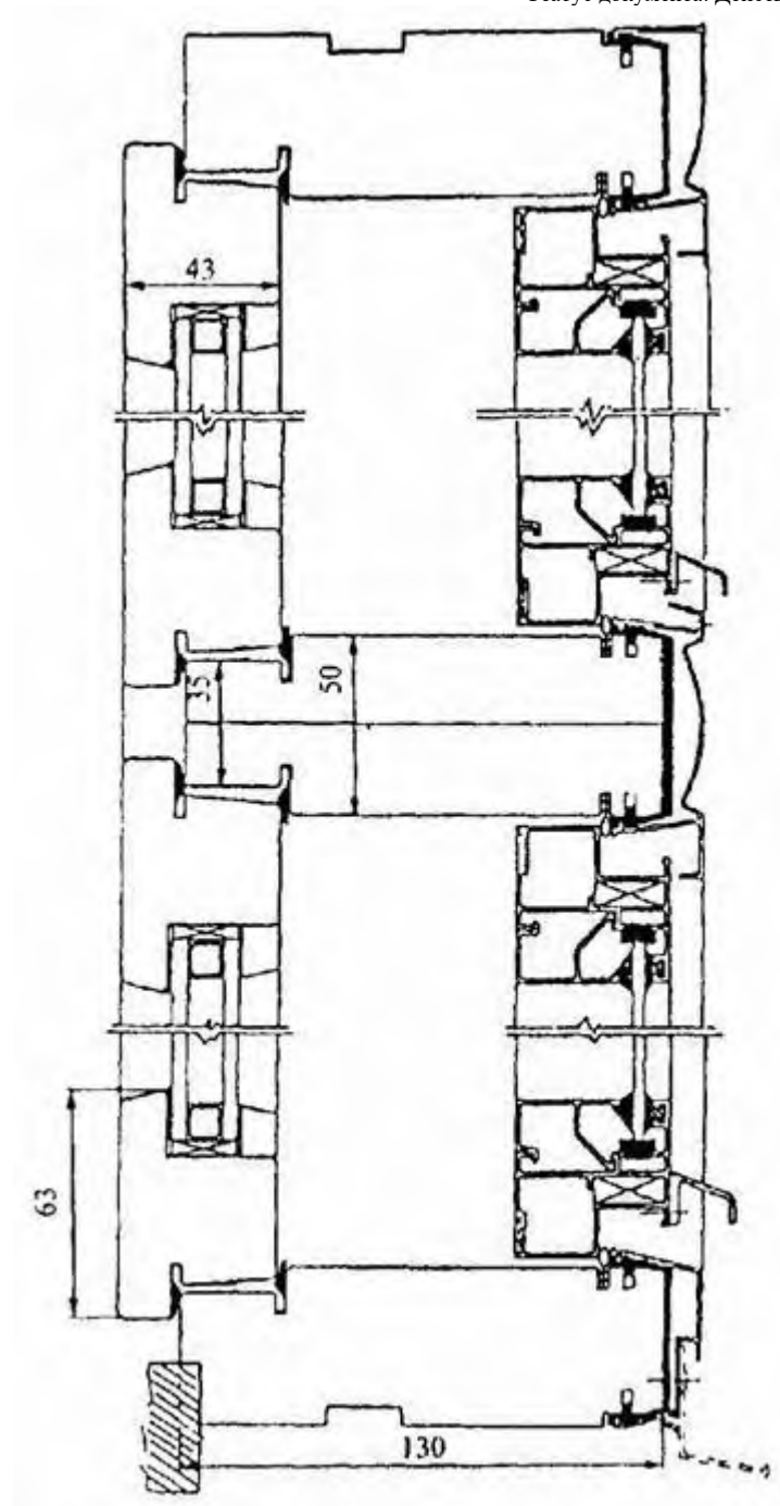
Рисунок 6 - Пример конструктивного решения оконного блока раздельной конструкции с листовым стеклом и стеклопакетом
