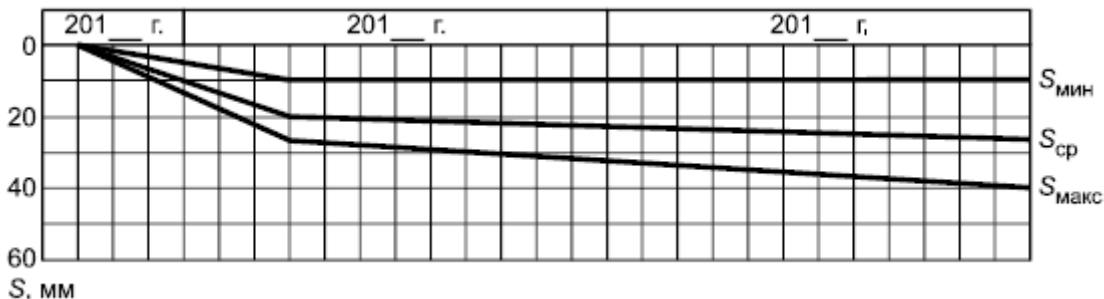
Рисунок Б.4 - График развития перемещений
