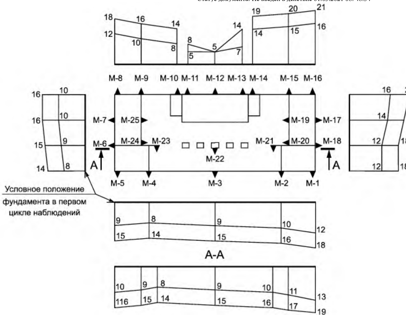
Рисунок Б.2 - План расположения марок и эпюры перемещений
