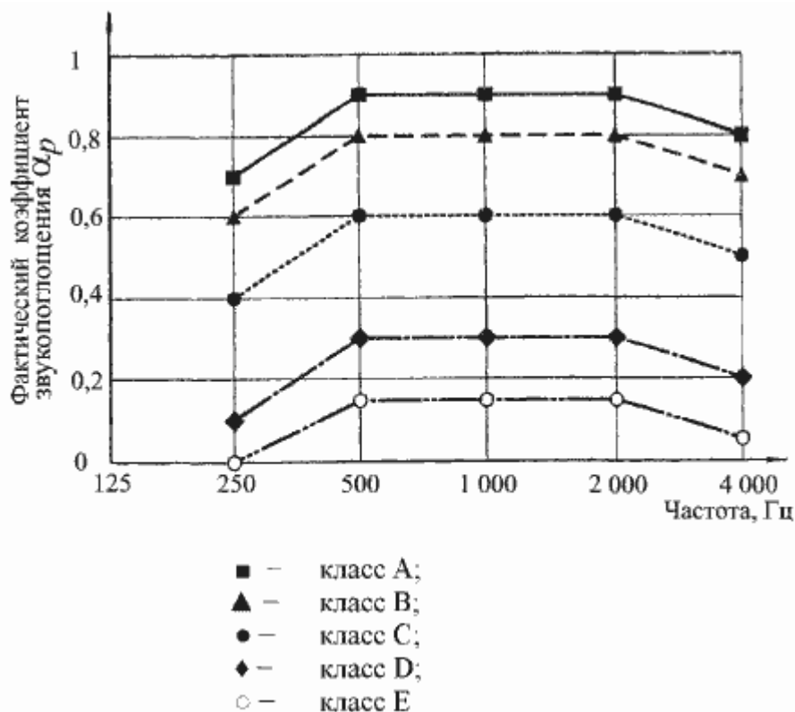
Рисунок 1 - Нормативные кривые, ограничивающие классы звукопоглощения
