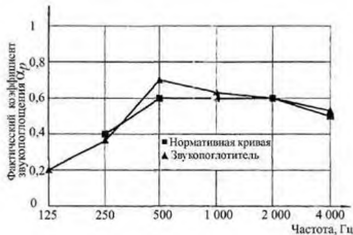
Рисунок В.3 - Пример определения индекса звукопоглощения \alpha_w ( \alpha_w = 0,60 )
