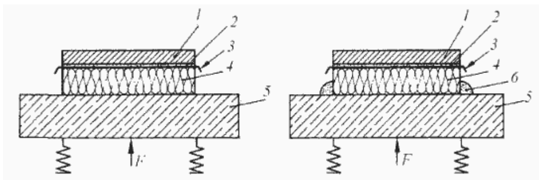
Рисунок Г.1 - Схема возбуждения нагружающей пластины. Измерение вибрации нагружающей пластины
