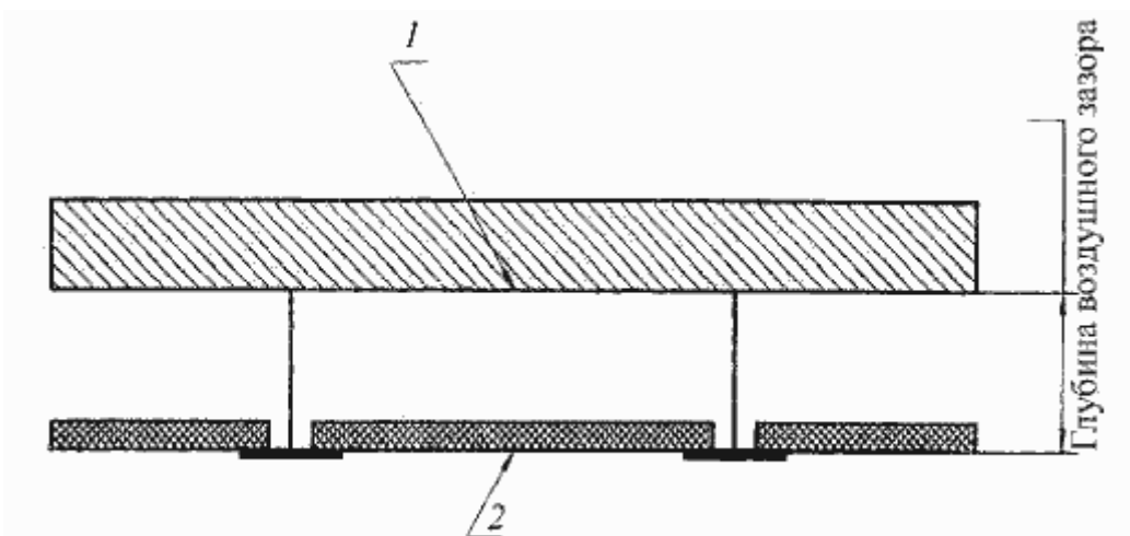
1 - поверхность помещения; 2 - звукопоглотитель
