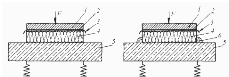
Рисунок Г.2 - Схема возбуждения нагружающей пластины. Измерение вибрации нагружающей пластины и основания
