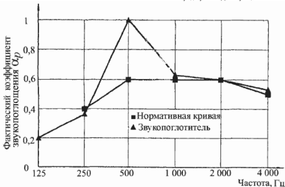
Рисунок В.4 - Пример определения индекса звукопоглощения с применением индикатора формы \alpha_w [ \alpha_w = 0,60 (М)]
