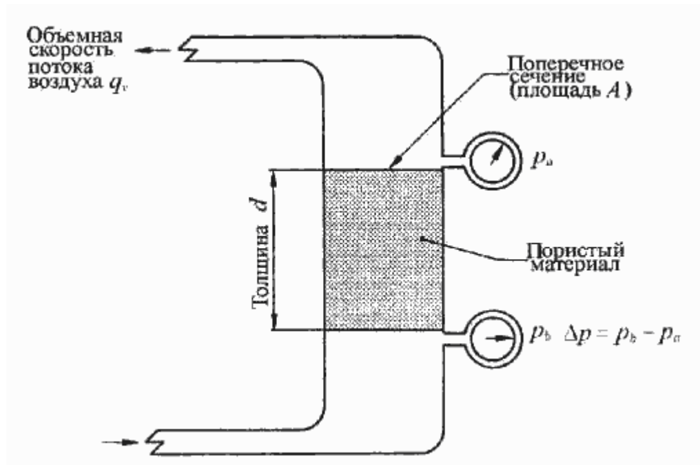
Рисунок Б.1 - Схема определения сопротивления продуванию постоянным потоком воздуха (метод А). Основной принцип
