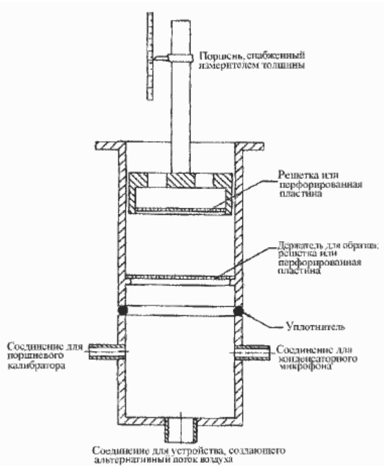
Рисунок Б.4 - Схема измерительной камеры, снабженная держателем для образца, изготовленного из волокнистого, сыпучего материала или материала плотной структуры (метод В)
