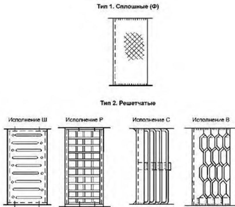
Рисунок 5 - Типы ступеней маршевых лестниц и настилов прямоугольных площадок
