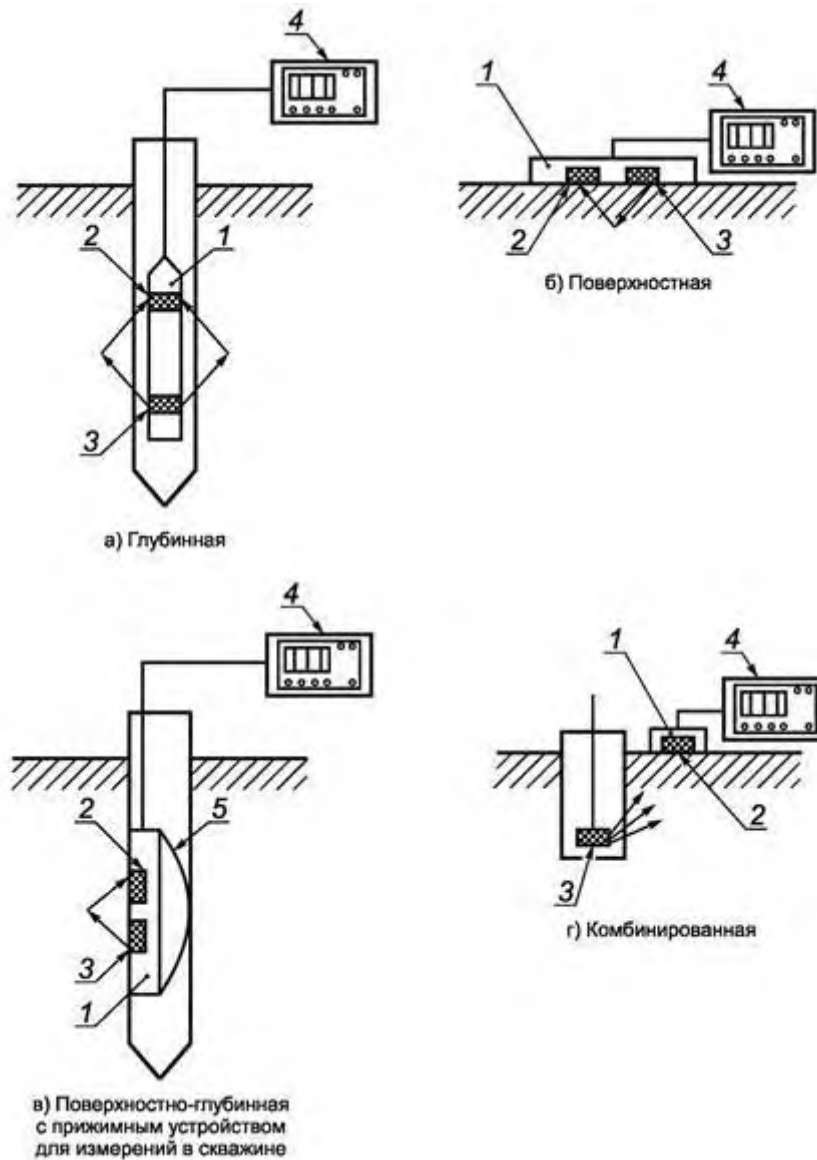
Рисунок 3 - Схемы измерений нейтронными влагомерами
