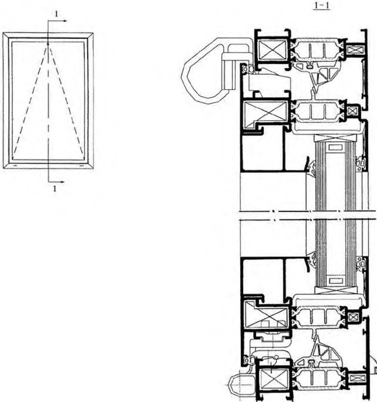
Рисунок 2 - Пример конструктивного решения оконного блока с откидным открыванием створки внутрь помещения
