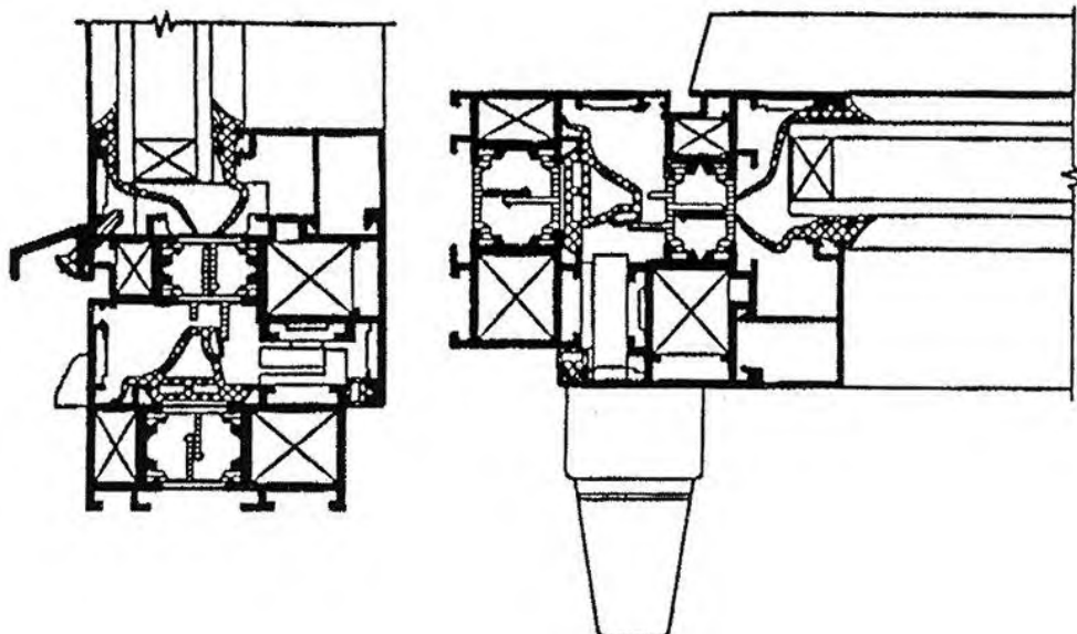
Рисунок 3 - Вариант конструктивного решения узлов притвора оконного блока с поворотно-откидным открыванием внутрь помещения
