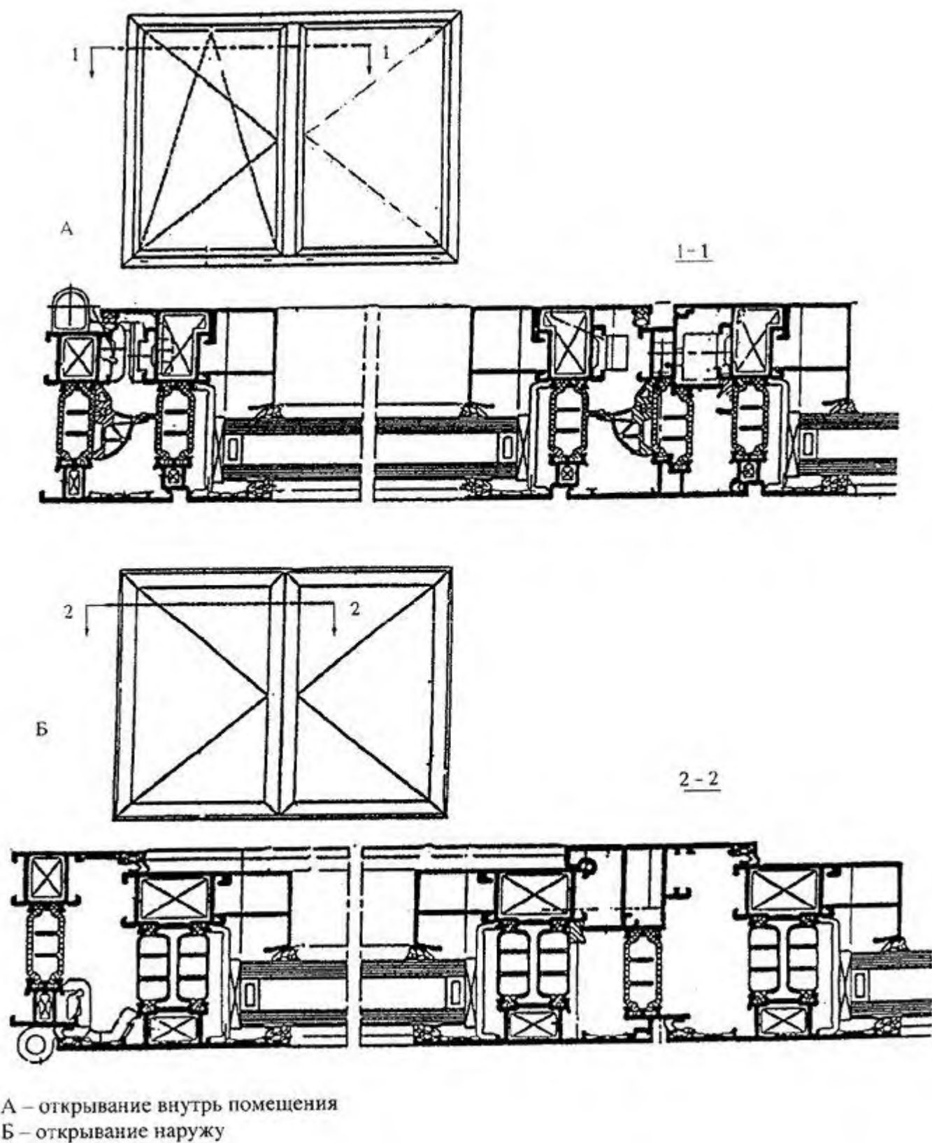
Рисунок 6 - Примеры конструктивного решения срединного притвора
