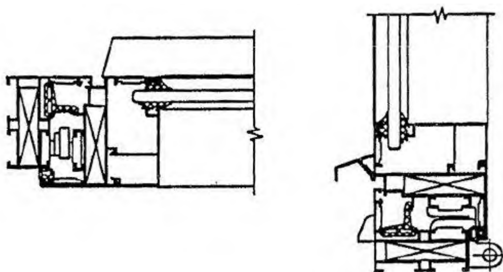
Рисунок 4 - Вариант конструктивного решения узлов притвора оконного блока с откидным открыванием внутрь помещения
