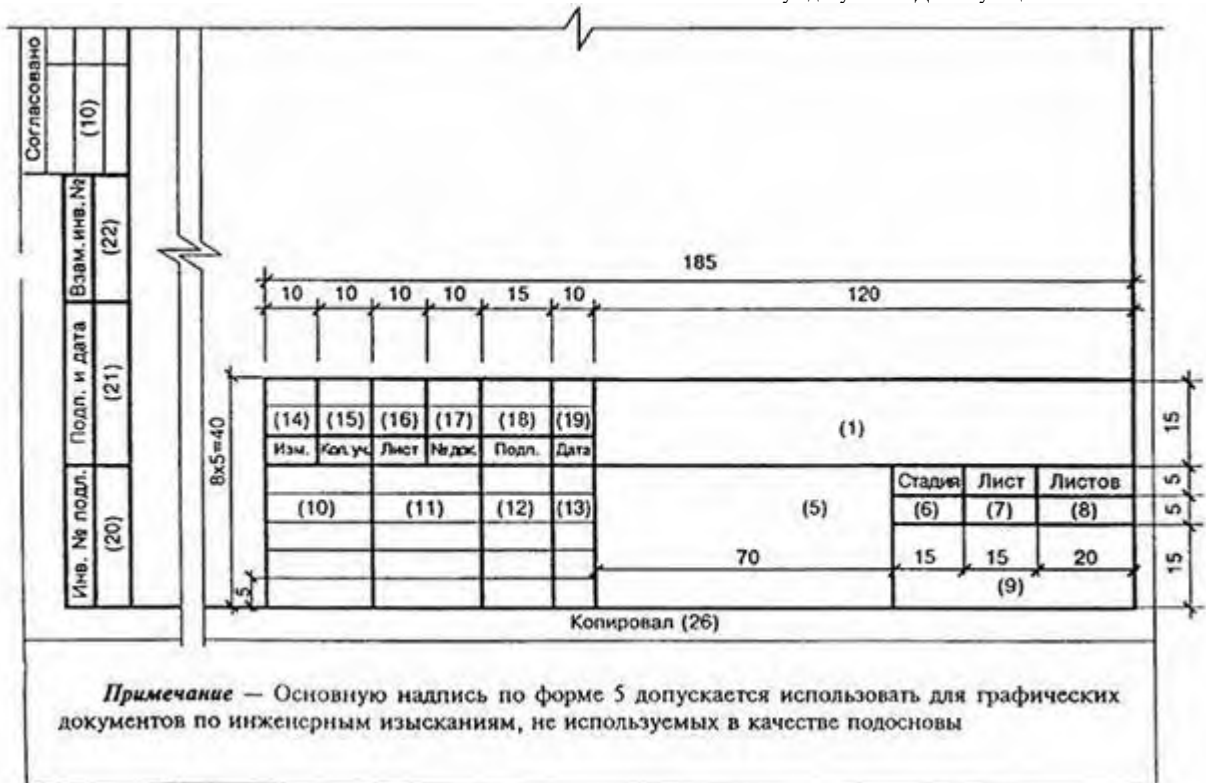
Форма 6 - Для чертежей строительных изделий и всех видов текстовых документов (последующие листы)
