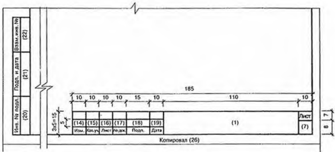
Форма 6 - Для чертежей строительных изделий и всех видов текстовых документов (последующие листы)
