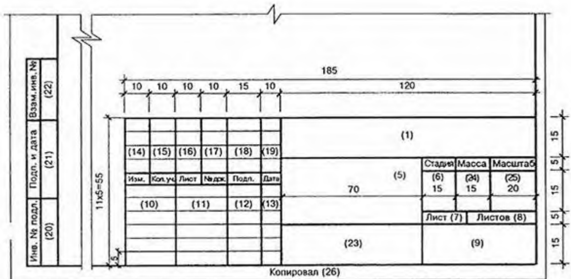
Форма 4 - Для чертежей строительных изделий (первый лист)
