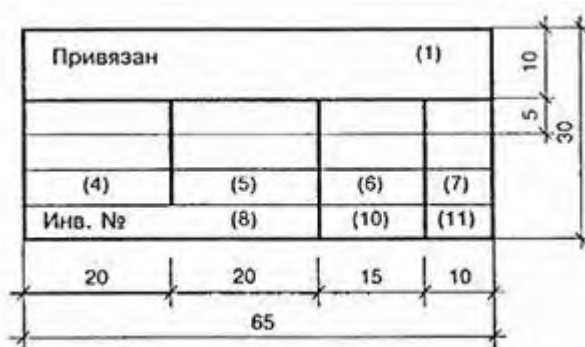
Форма 13 - Штмп привязки (последующие листы)
