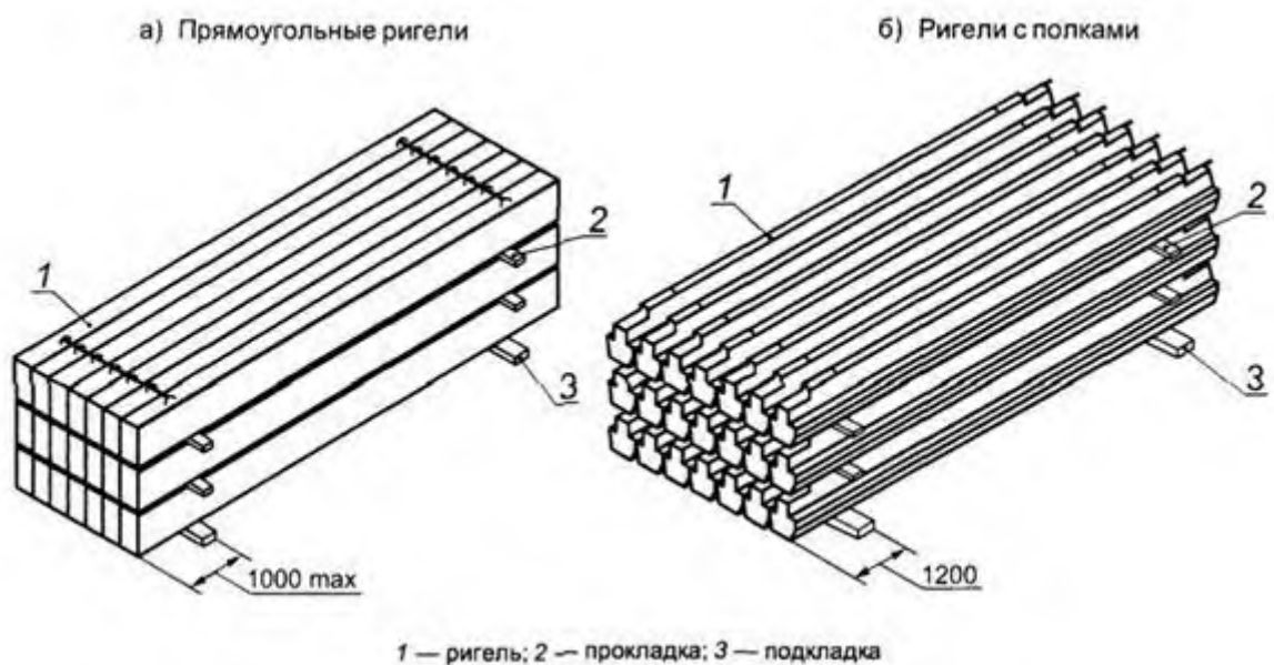
«Рисунок 1 - Складирование ригелей»
