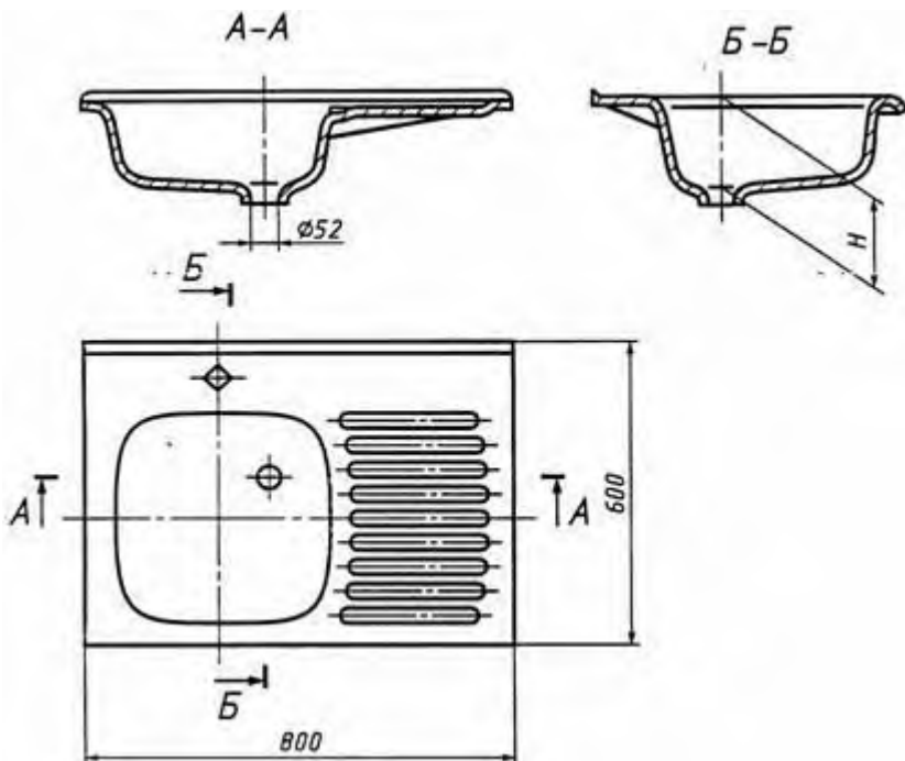
Рисунок 8 - Мойка чугунная эмалированная со сливной полкой
