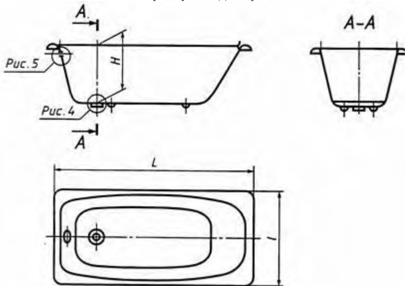
Рисунок 1 - Ванна чугунная эмалированная
