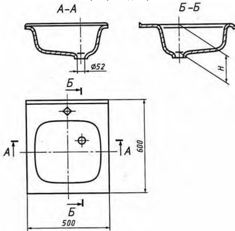
Рисунок 7 - Мойка чугунная эмалированная с одной чашей
