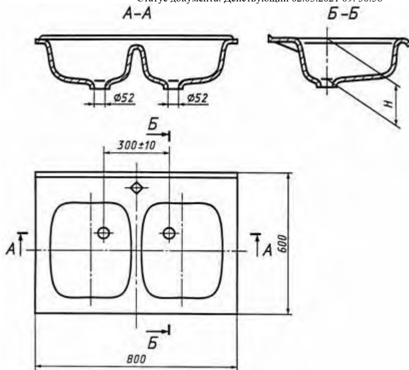
Рисунок 9 — Мойка чугунная эмалированная с двумя чашами
