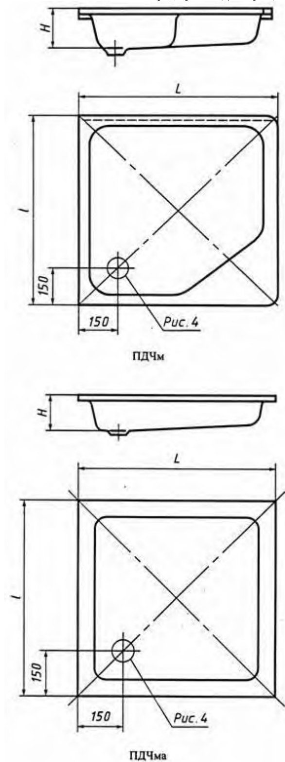
Рисунок 3 - Поддон душевой чугунный эмалированный мелкий
