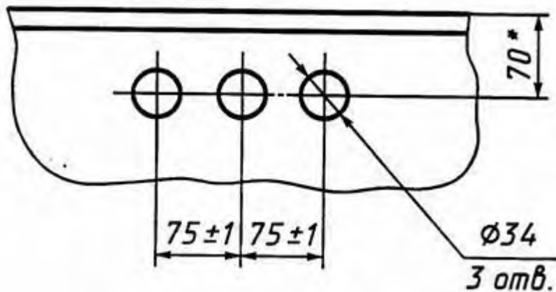
б) для смесителя со щеткой
