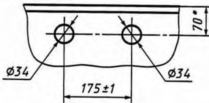
а) для центрального смесителя
