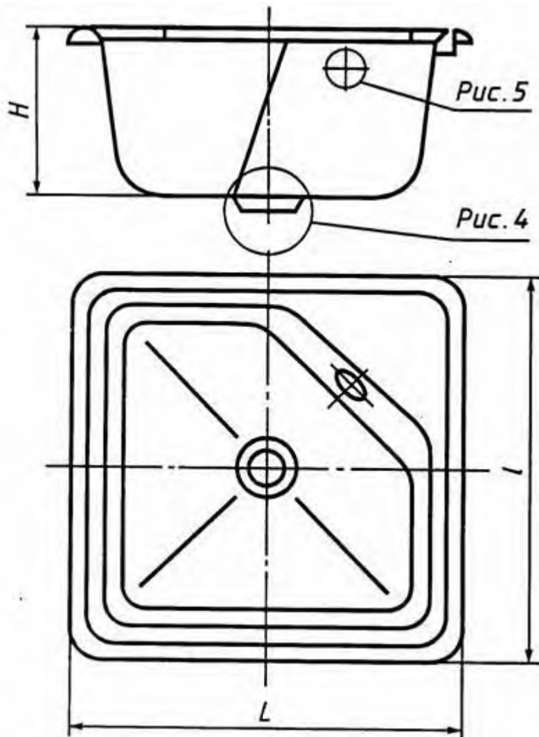
Рисунок 2 - Поддон душевой чугунный эмалированный глубокий
