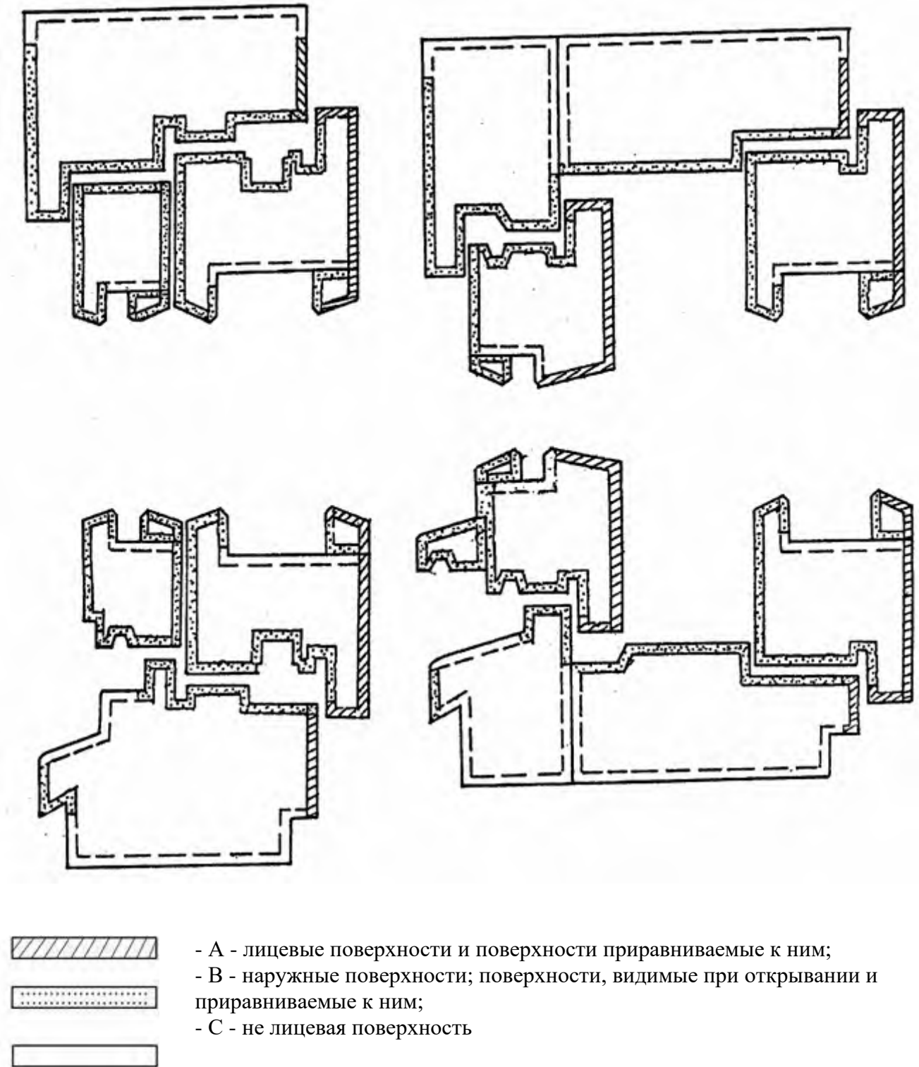
Рисунок 11 - Примеры определения видов поверхностей деталей
