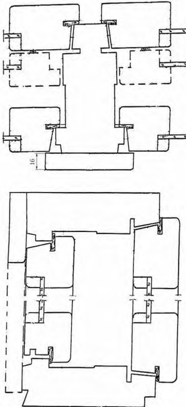
Рисунок 7 - Пример раздельной конструкции оконного блока с двойным остеклением (бруски коробки имеют универсальный профиль, что позволяет устанавливать дополни- тельную створку и преобразовывать конструкцию в раздельно-спаренную)
