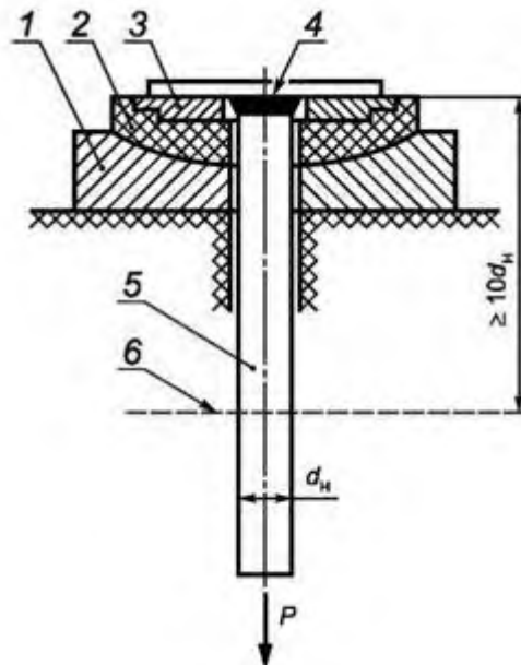
Рисунок 4 - Схемы испытаний крестообразных соединений на срез
