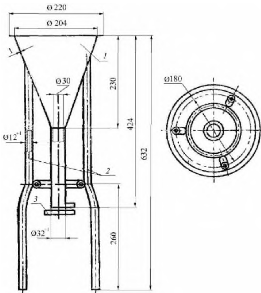
1 - воронка; 2 - опоры; 3 - заслонка
