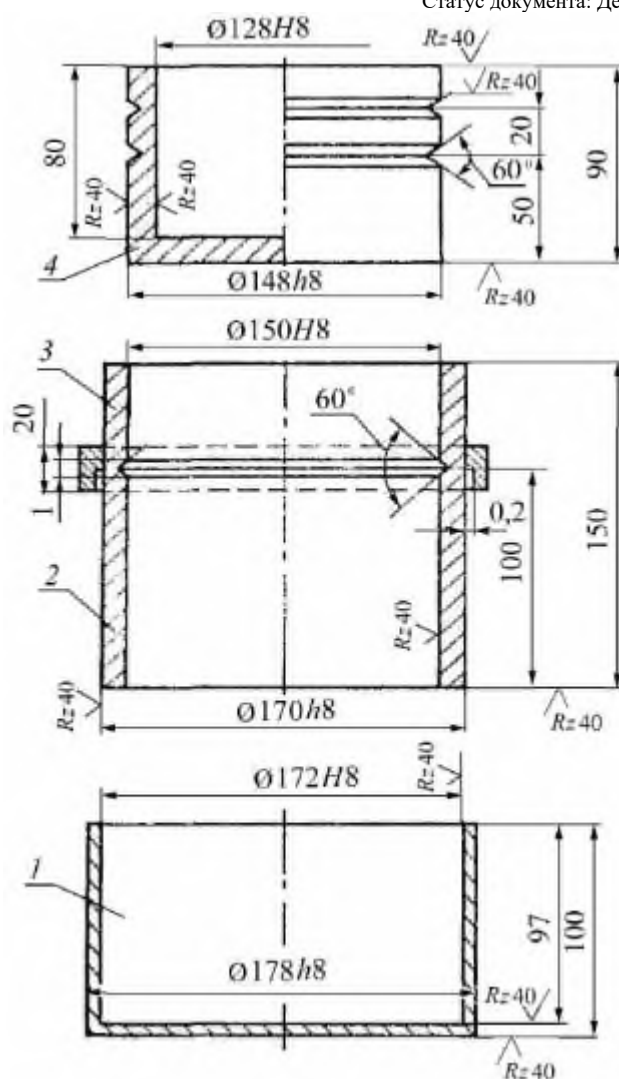
1 - поддон; 2 - цилиндр; 3 - приставка; 4 - пуансон
