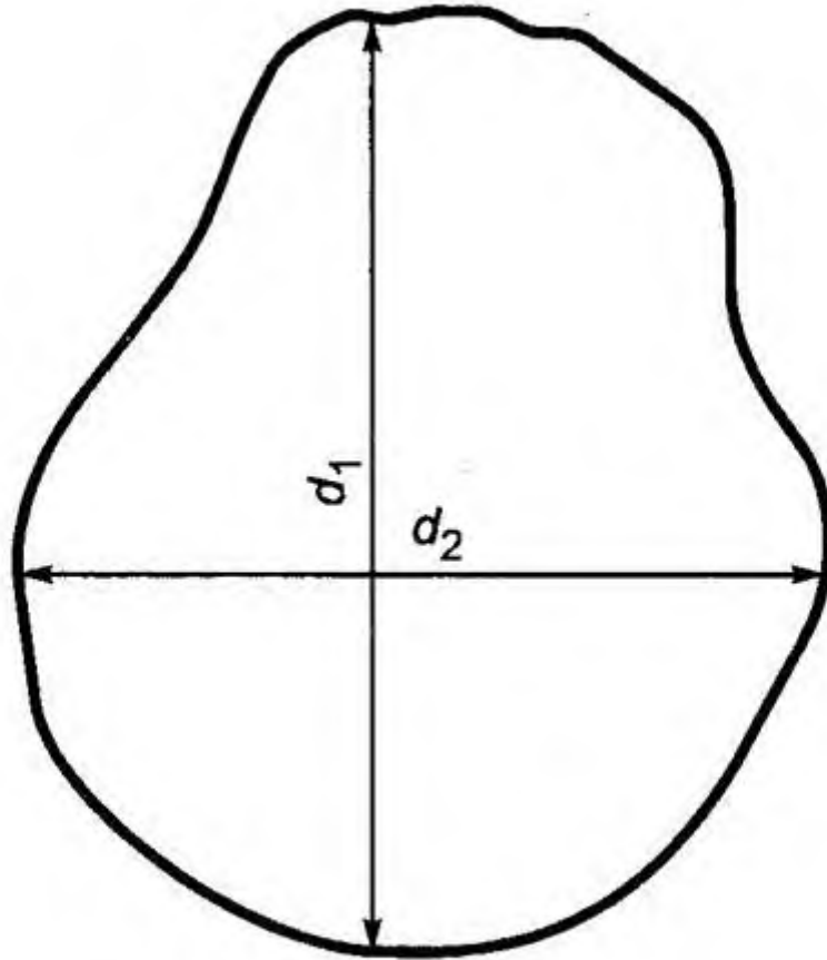
Рисунок 7 — Измерение расплыва бетонной смеси
