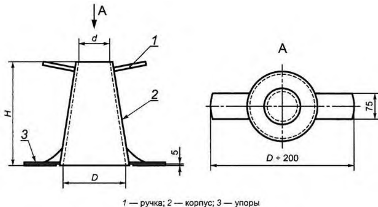
Рисунок 1 — Конус для определения подвижности
