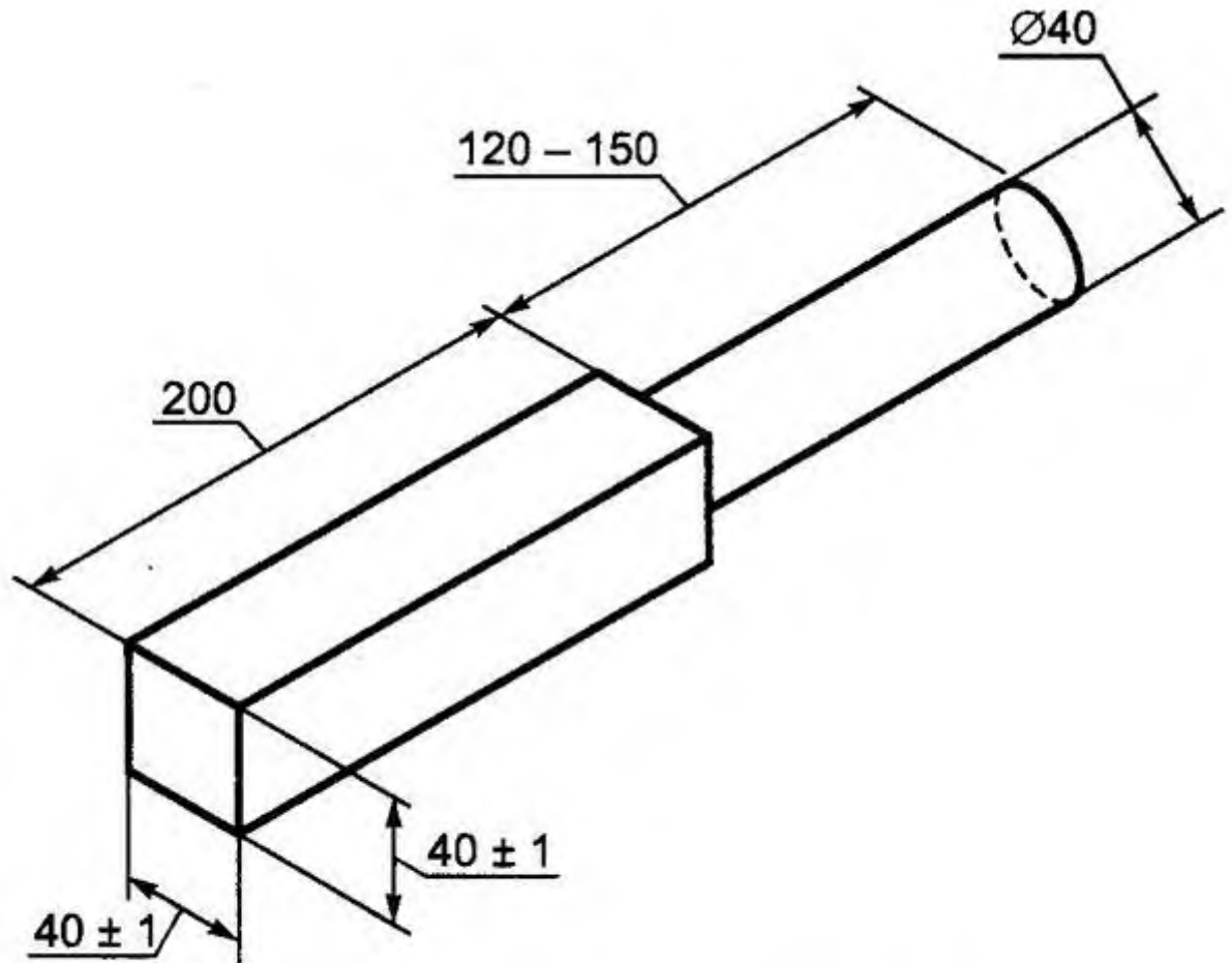
Рисунок 6 — Уплотняющий брус
