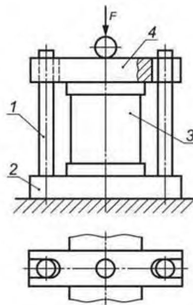
Рисунок И.2 - Схема кондуктора
