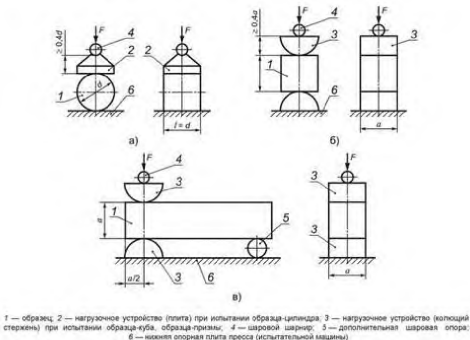
Рисунок И.1 - Схема устройств для испытаний на растяжение при раскалывании
