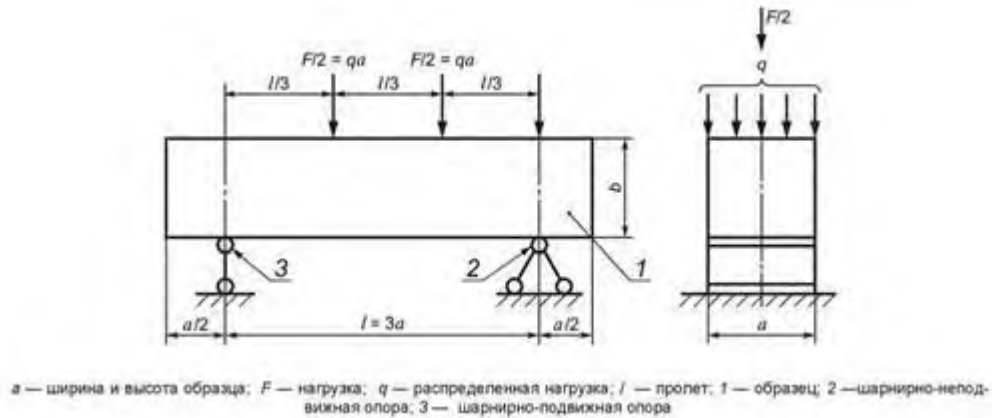
Рисунок 2 - Схема испытания на растяжение при изгибе
