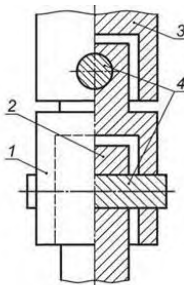
Рисунок К.4 - Схема саморегулируемого зажима
