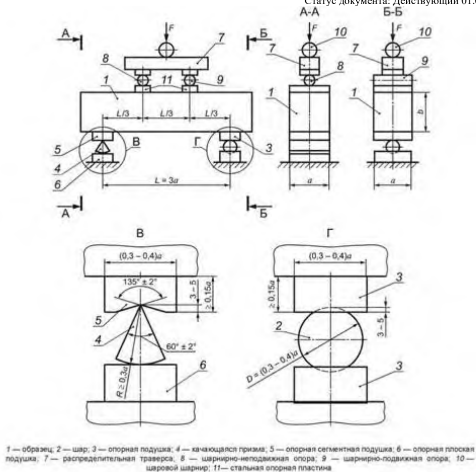
Рисунок Ж.1 - Схема устройств для испытания на растяжение при изгибе
