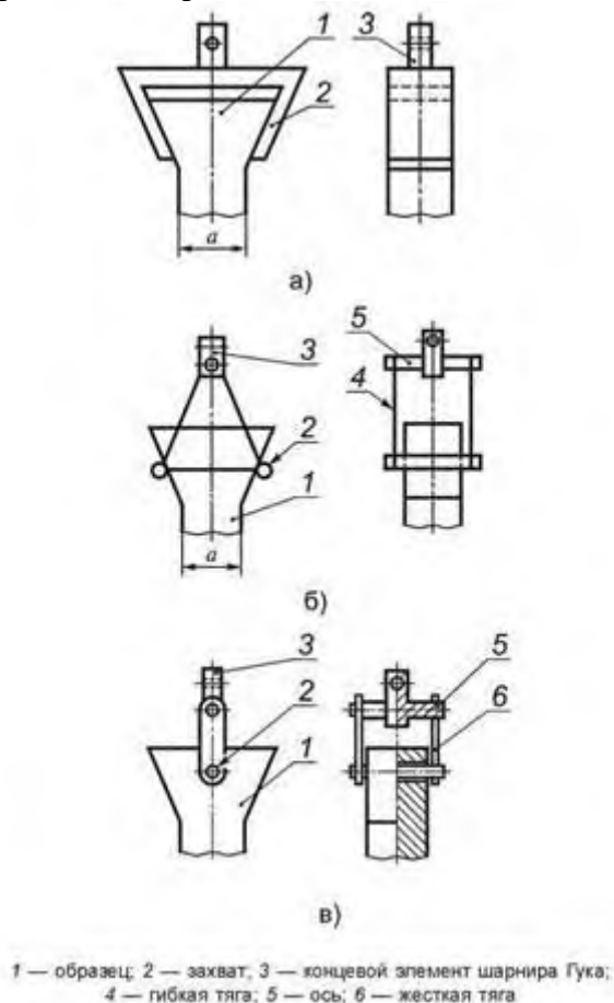
Рисунок К.1 - Схемы захватов для крепления образца с галтелями
