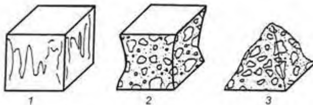
Рисунок Е.1 — Удовлетворительные разрушения образцов-кубов
