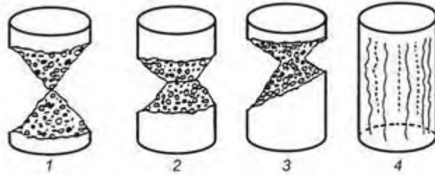
Рисунок Е.3 — Удовлетворительные разрушения образцов-цилиндров
