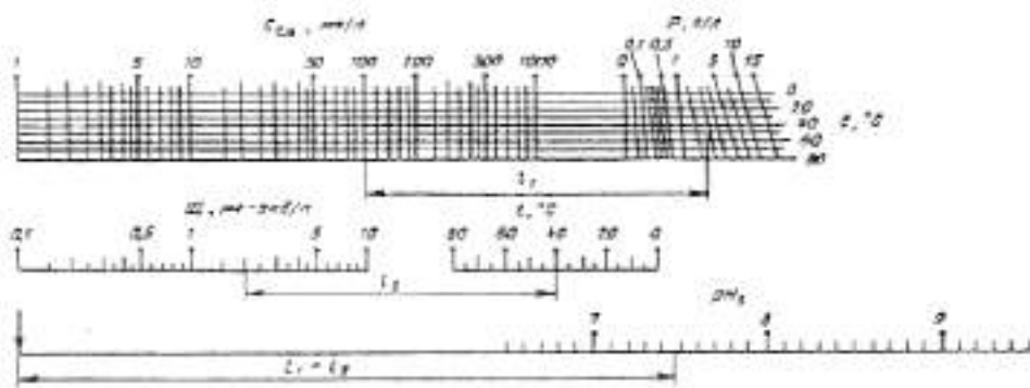
Рис. 1. Номограмма для определения pH насыщения воды карбонатом кальция ( pH_s )
