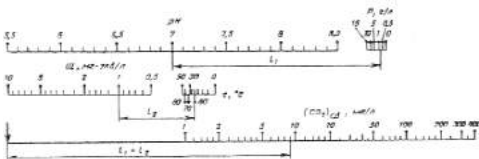
Рис. 2. Номограмма для определения концентрации свободной двуокиси углерода в природной воде (или pH)
