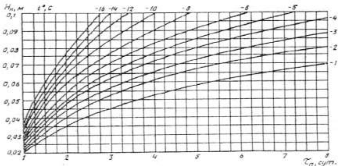
Рис. 7. Зависимость глубины промораживания слоя осадка от среднесуточной температуры воздуха и продолжительности промораживания
