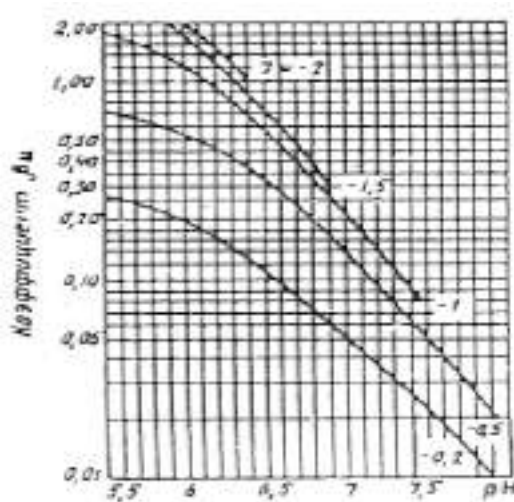
Рис. 4. Номограмма для определения коэффициента \beta_{и} при расчете дозы щелочи
