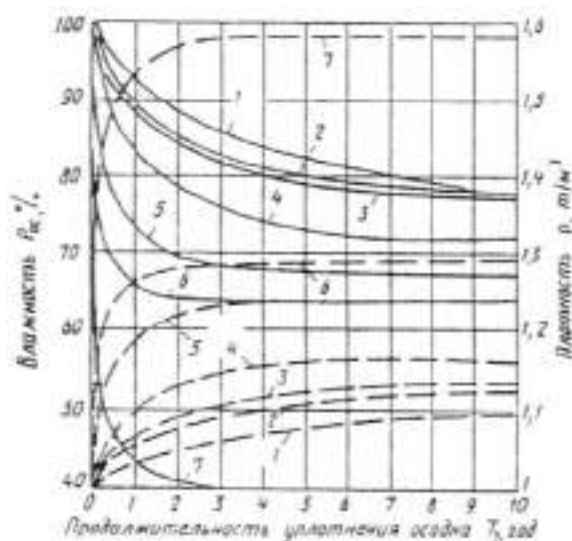
Рис. 1. Средние значения влажности и плотности осадка станций осветления и обесцвечивания воды при многолетнем уплотнении
