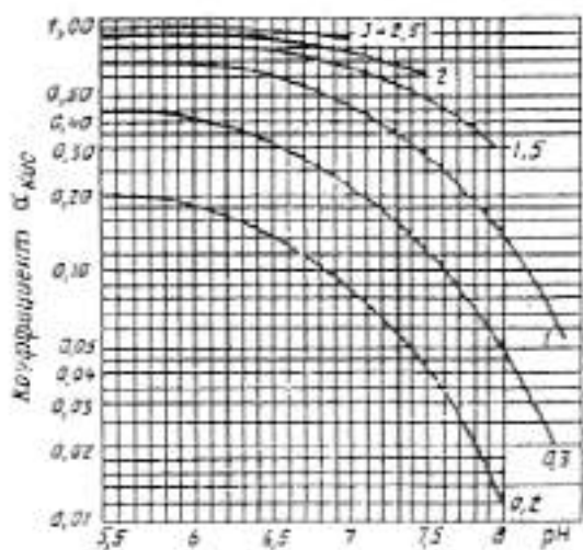
Рис. 3. Номограмма для определения коэффициента \alpha_{кис} при расчете дозы кислоты
