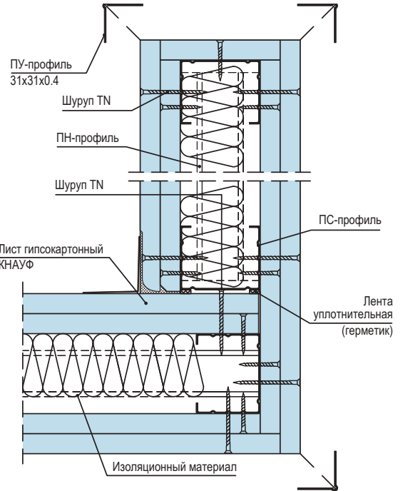
Рисунок 14 – Выполнение угла и обрамление проема в перегородках по типу C12
