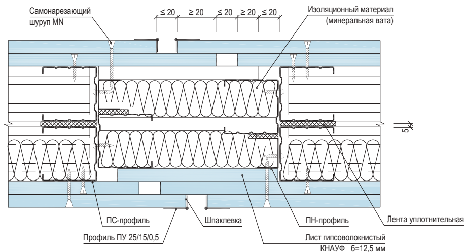
Рисунок 7 – Устройство деформационного шва в перегородках по типу С365
