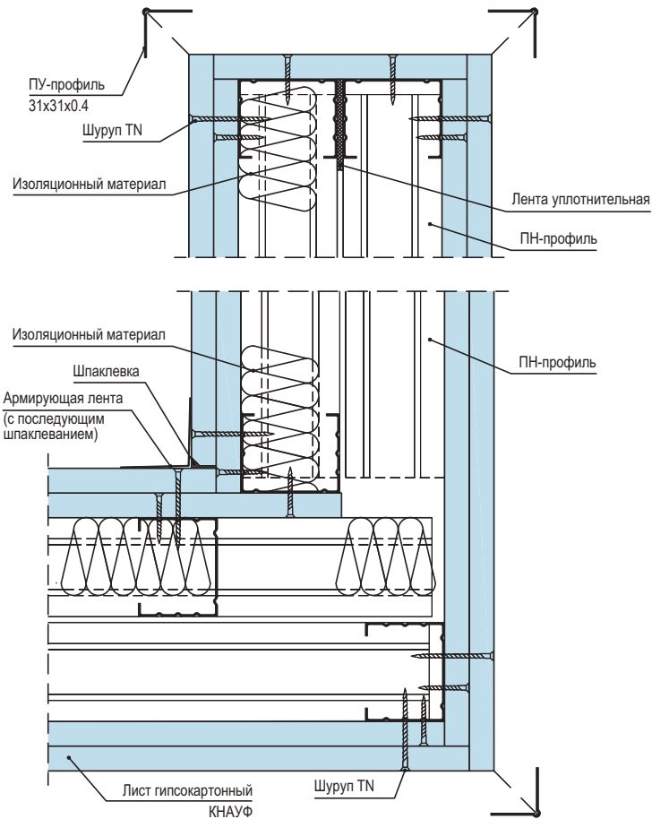
Рисунок 15 – Выполнение угла в перегородках по типу C113
