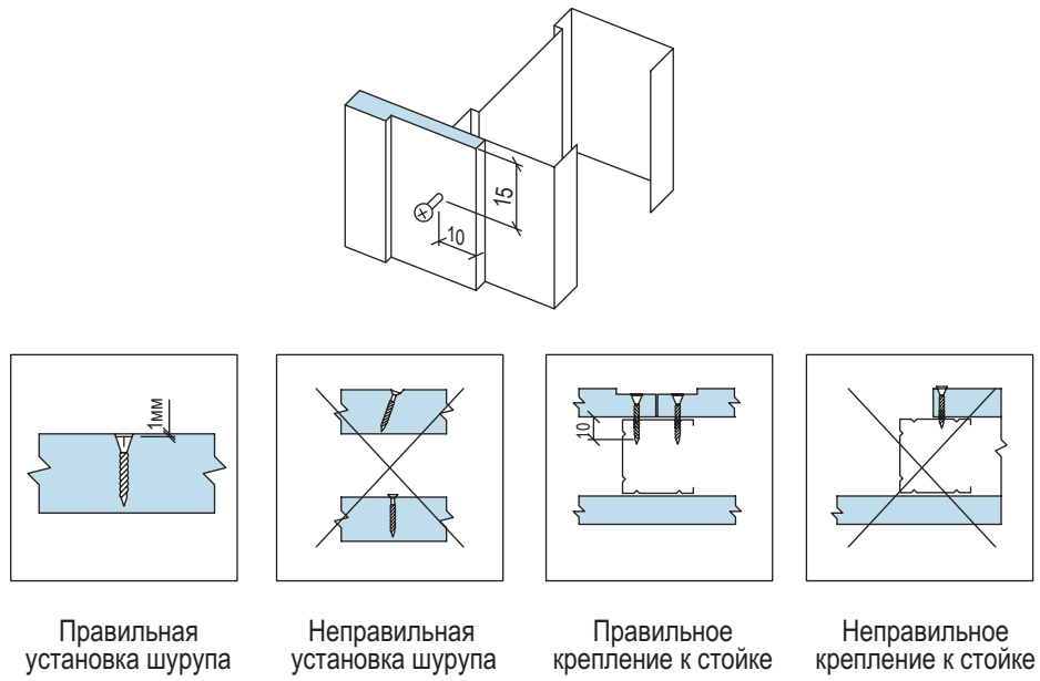
Рисунок 7 – Крепление ГВЛ к стойке.
