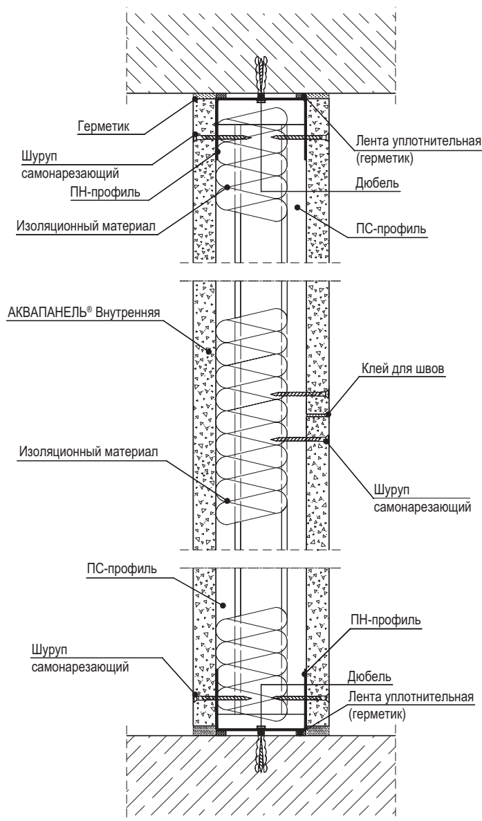
Рисунок 4 – Вертикальный разрез перегородки C381
