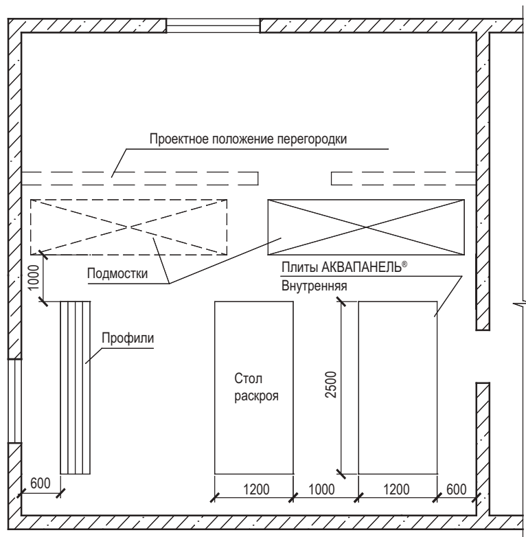
Рисунок 1 – Схема организации рабочего места
