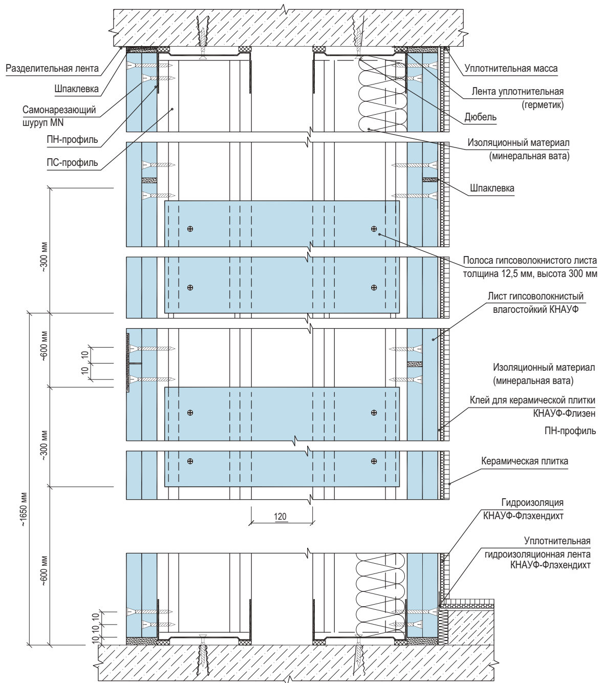
Рисунок 13 – Вертикальный разрез перегородки по типу С366.
