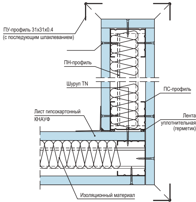
Рисунок 13 – Выполнение угла и обрамление проема в перегородках по типу C11
