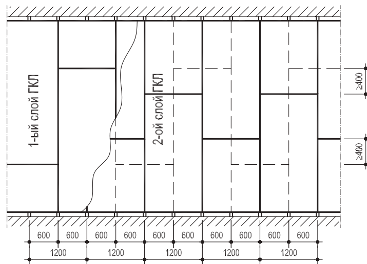
Рисунок 12 – Схема установки гипсокартонных листов 1-го и 2-го слоев
