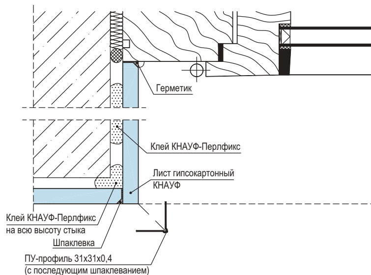
Рисунок 9 – Выполнение обрамления оконного (дверного) проема
