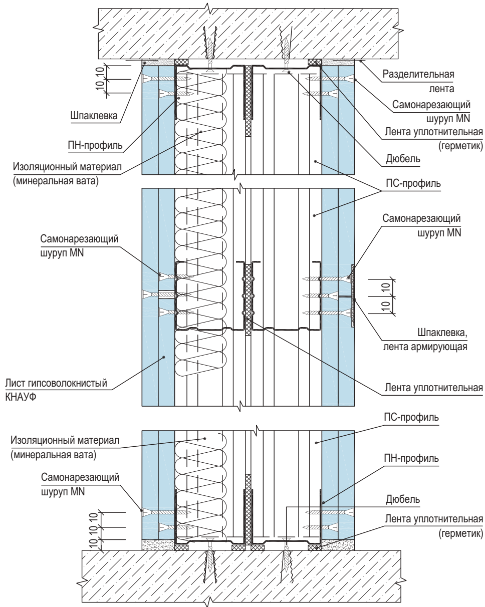
Рисунок 12 – Вертикальный разрез перегородки по типу C365.
