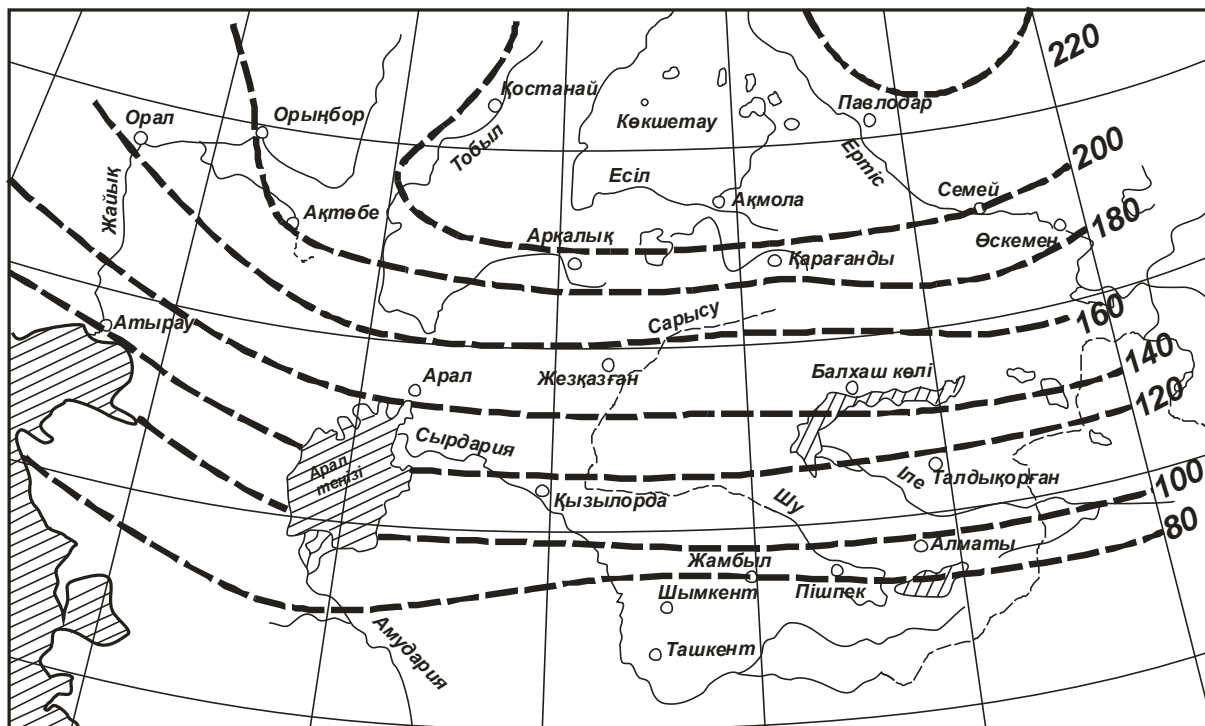
Сурет Г.1 – Қазақстан бойынша топырақтардың нормативтік тоңдану тереңдіктерінің арасызықтары
