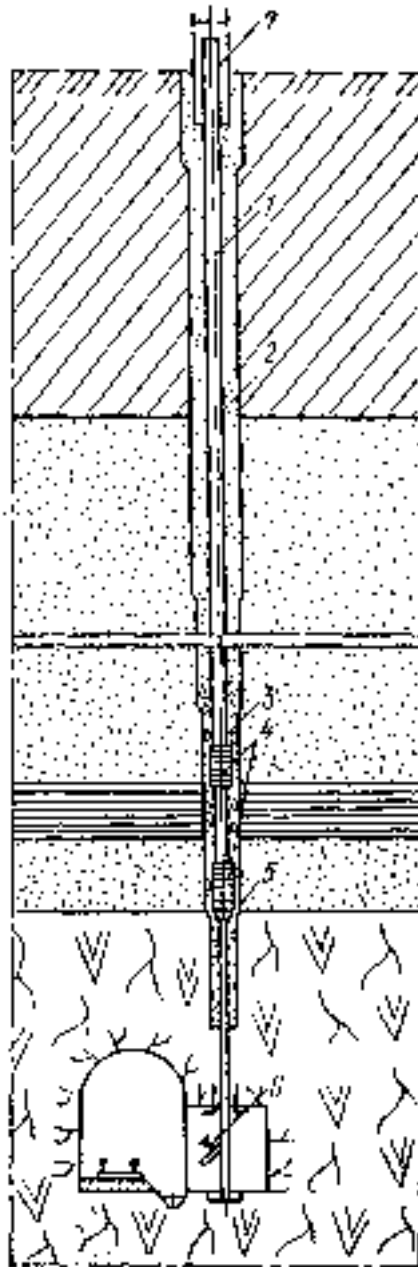
Рис. 38. Сквозной фильтр
