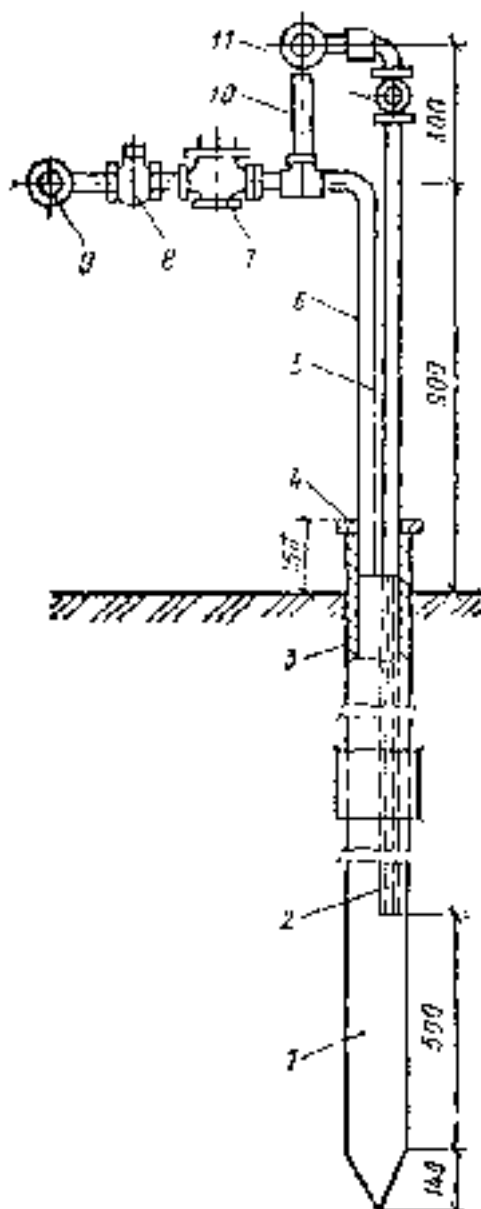
Рис. 78. Замораживающая колонка
