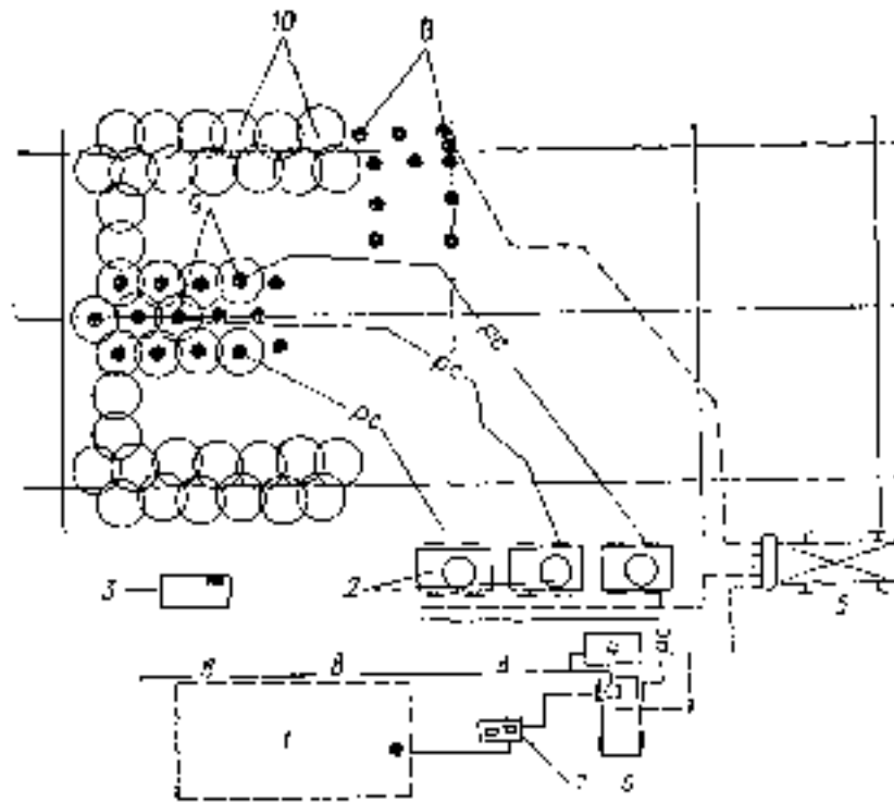
Рис. 66. Схема организации работ по закреплению грунтов через иньекторы
