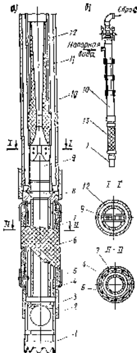
Рис. 51. Эжекторный иглофильтр
