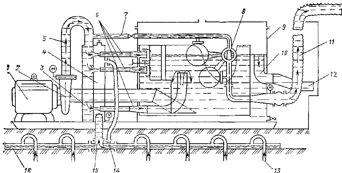
Рис. 49. Схема насосной установки УВВ-3
