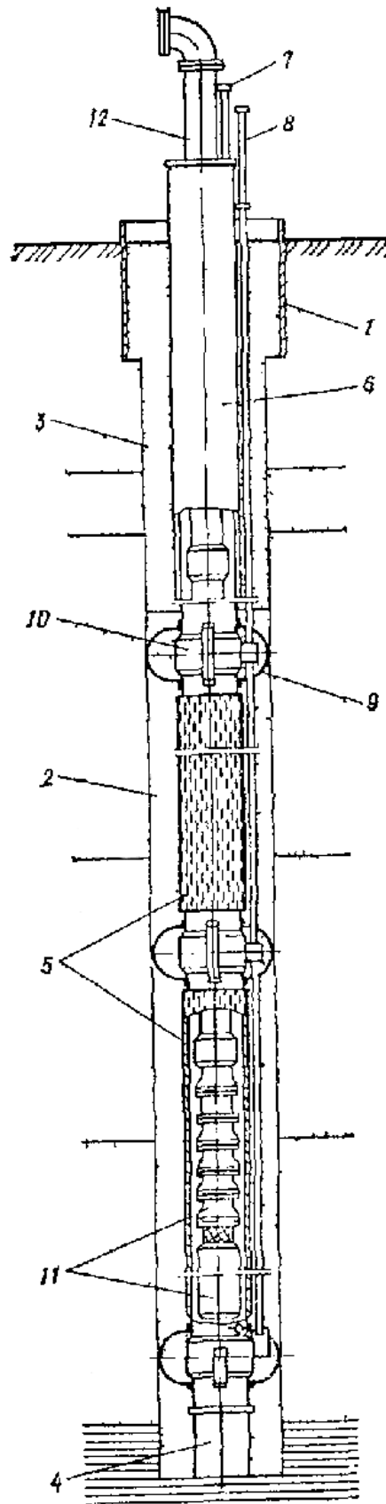
Рис. 33. Открытая скважина, оборудованная насосом
