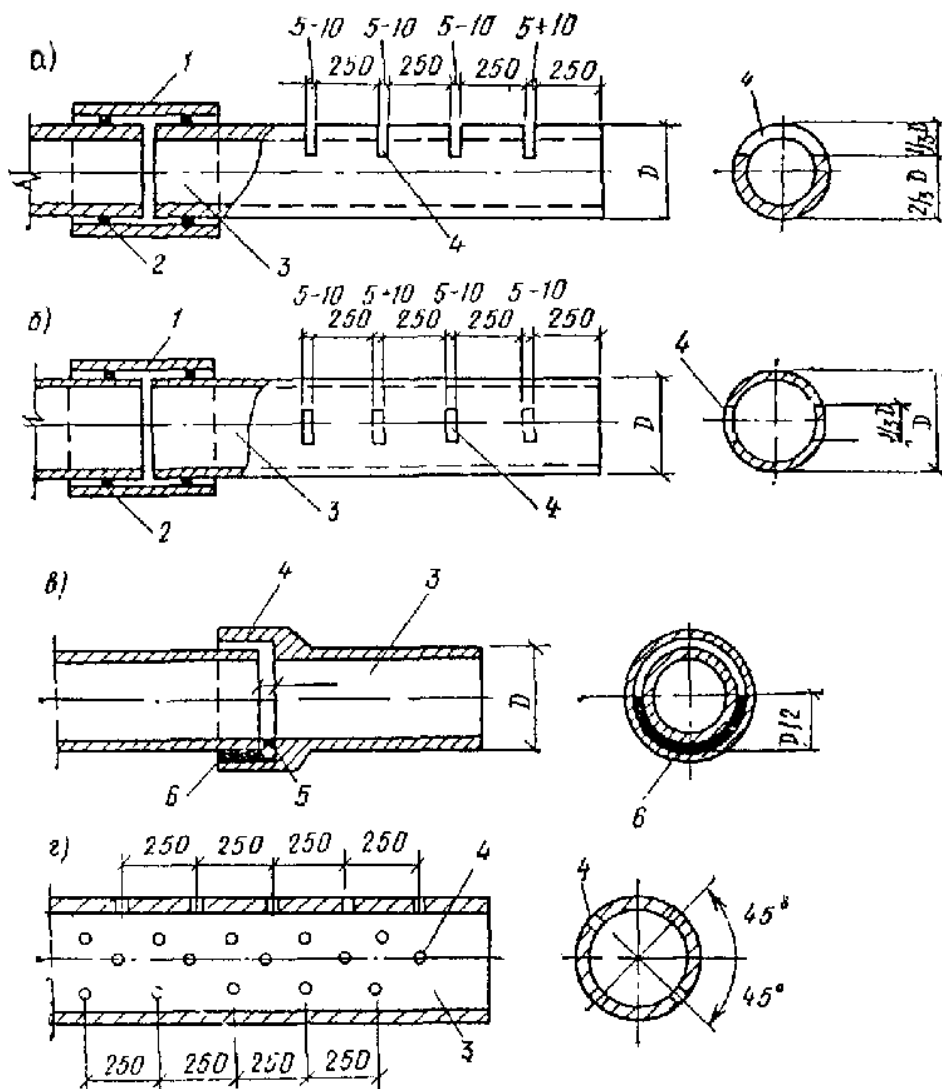
Рис. 28 Водоприемные отверстия в дренажных трубах
