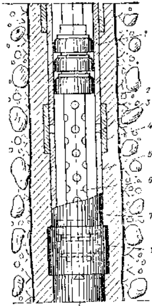
Рис. 62. Схема манжетно-тампонного иньектора
