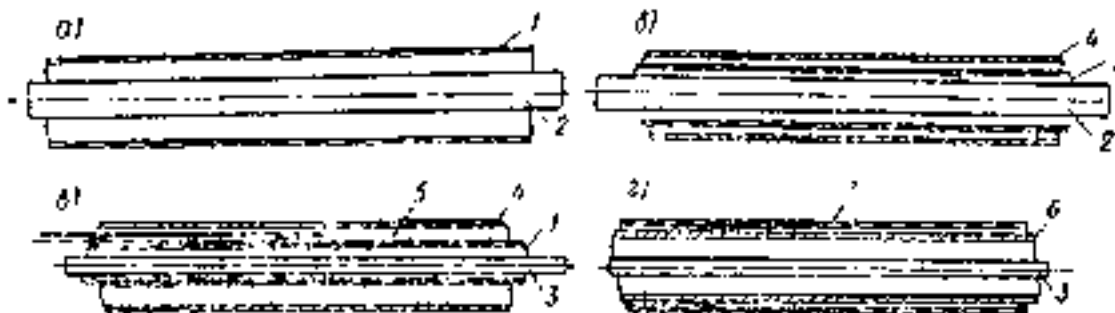
Рис. 41. Схемы устройства горизонтальных скважин
