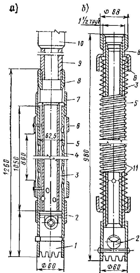
Рис. 48. Конструкция иглофильтров
