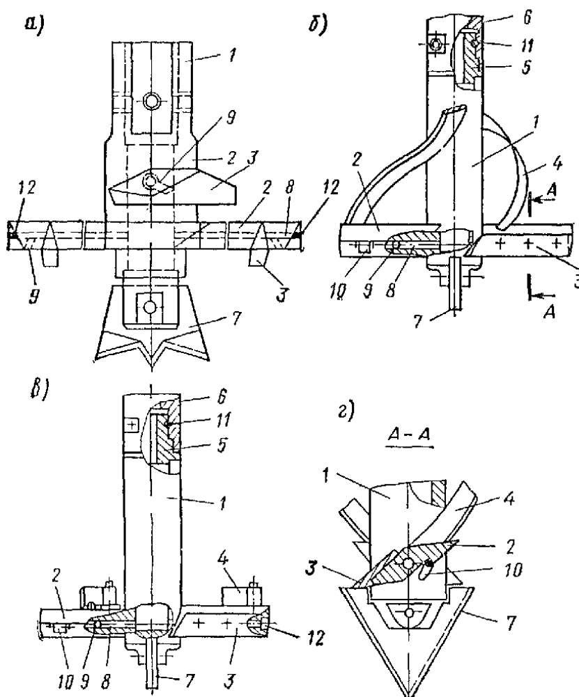
Рис. 71. Схемы буросмесителей
