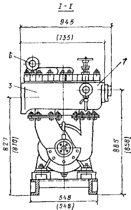
Рис. 47. Насосная установка ЛИУ-6Б
