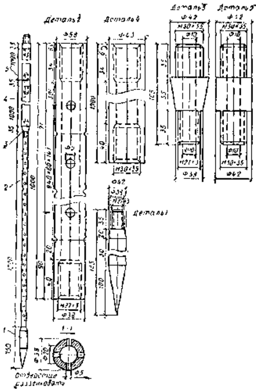
Рис. 59. Конструкция забивного инъектора переменного сечения для силикатизации просадочных лессовых грунтов
