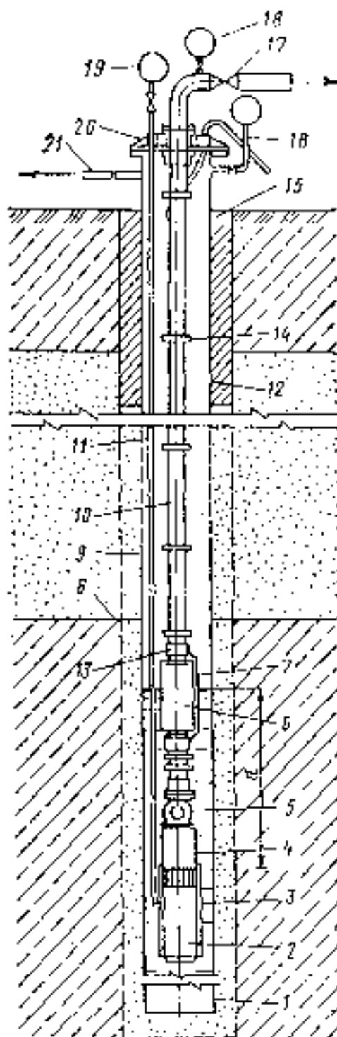
Рис. 40. Вакуум-скважина
