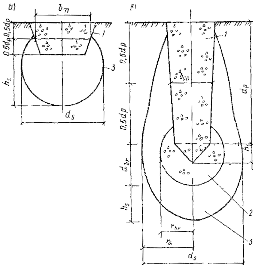
Рис. 1. Фундаменты в вытрамбованных котлованах
