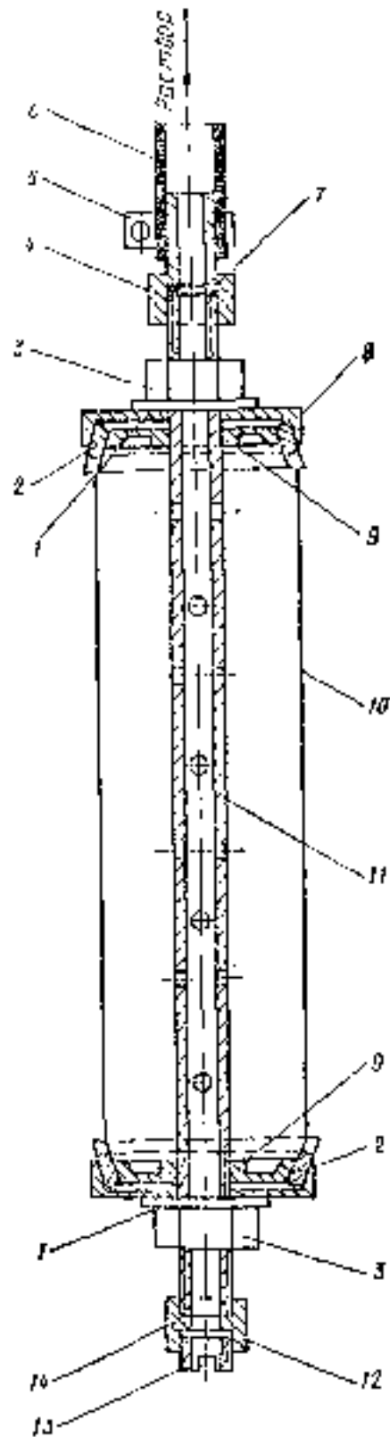
Рис. 60. Иньектор - тампон гидравлический, одинарный для силикатизации просадочных лёссовых грунтов в скважинах
