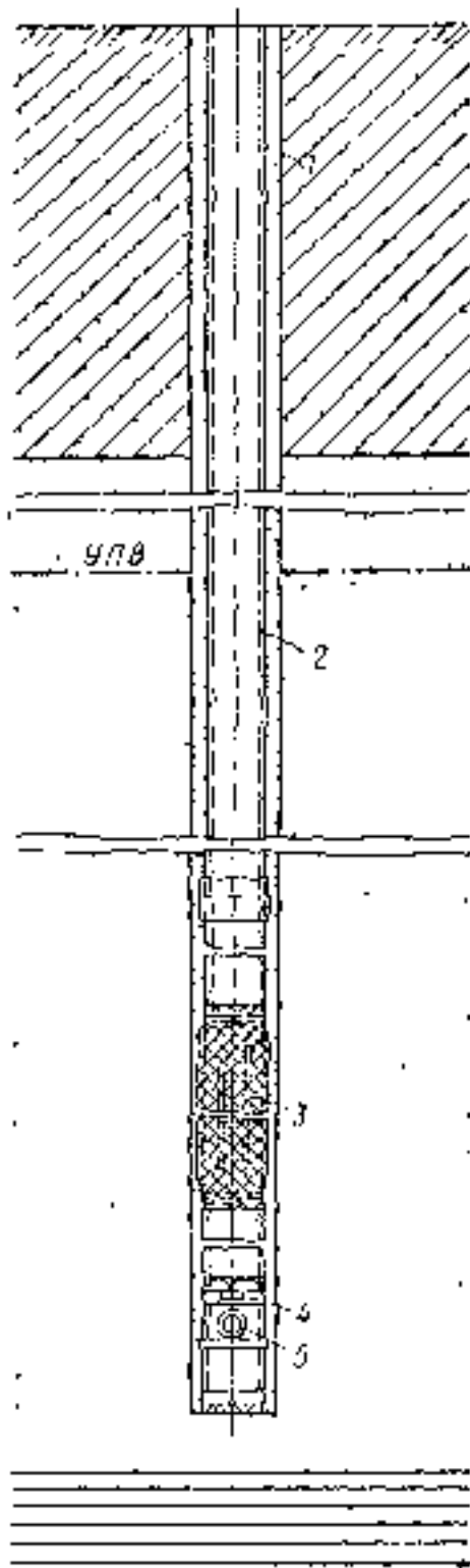
Рис. 54. Наблюдательная скважина
