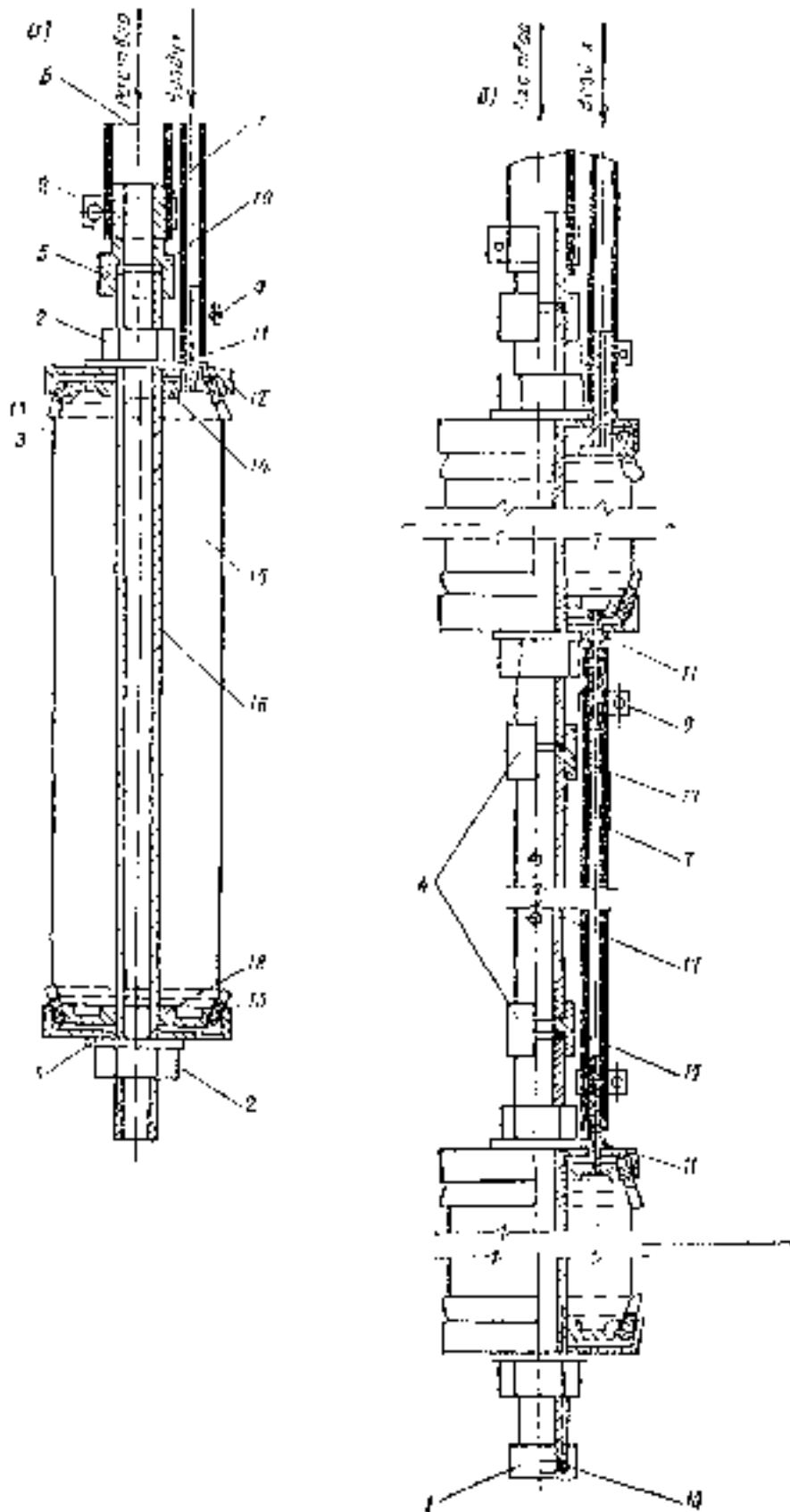
Рис. 61. Инъекторы - тампоны пневматические
