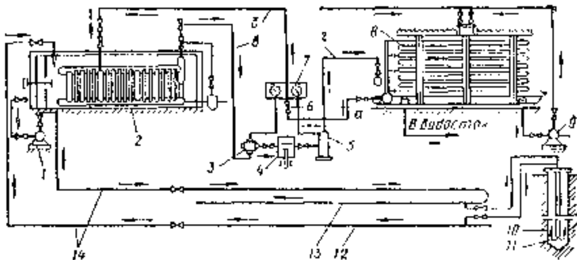
Рис. 76. Схема работы замораживающей станции
