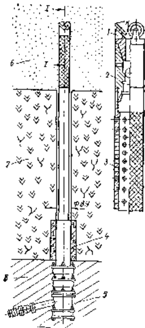
Рис. 37. Восстающая скважина
