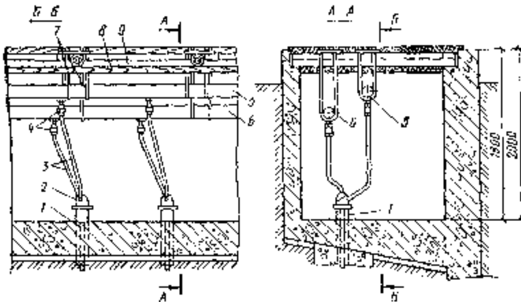
Рис. 77. Расположение рассольных коммуникаций в форшахте
