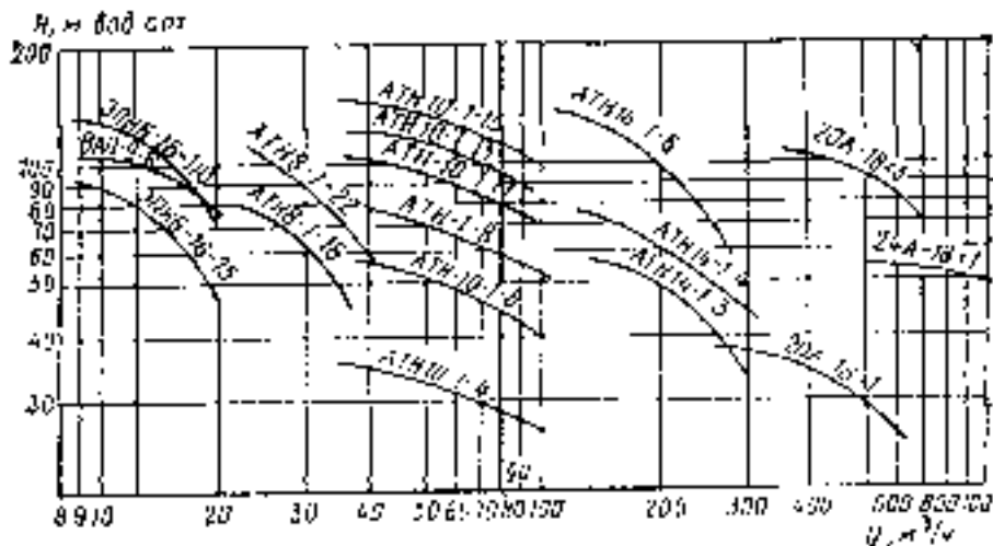
Рис. 30. Характеристики насосов типа А, АП, АТН, АПН
