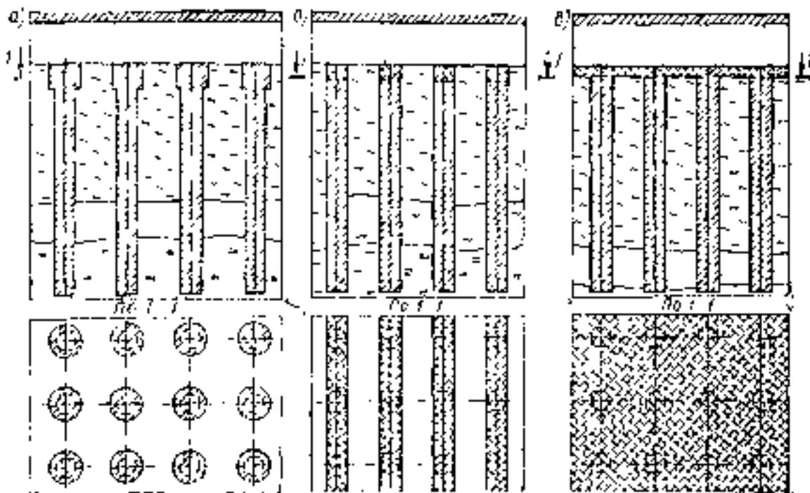
Рис. 72. Схемы устройства оголовков илоцементных свай в виде:
